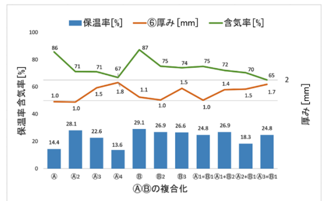
図3 改質リネン④⑥の複合化と保温率の関係
