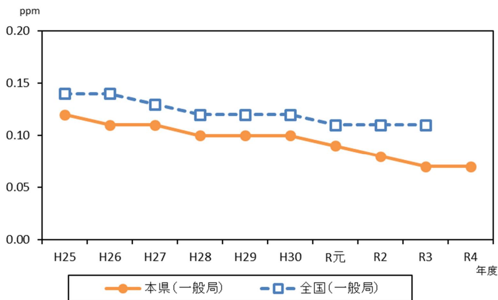
図2-7 本県及び全国の非メタン炭化水素濃度（年平均値）の推移
