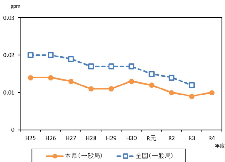
図 2-10 本県及び全国の浮遊粒子状物質（年平均値）の推移
