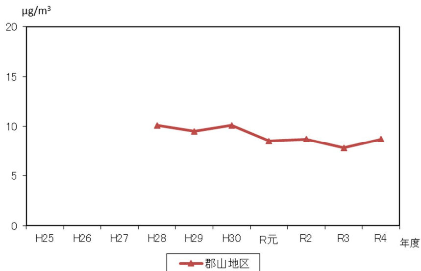
図 2-14 微小粒子状物質（年平均値）の経年変化
