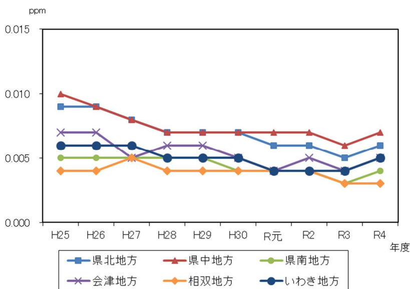
図 2-9 地方別の二酸化窒素濃度（年平均値）の推移
