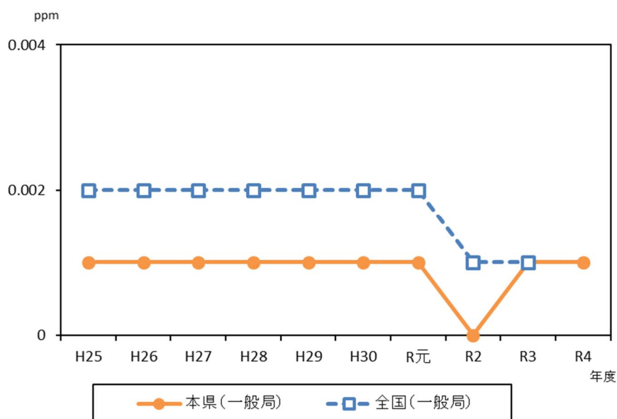
図 2-12 本県及び全国の二酸化硫黄濃度（年平均値）の推移
