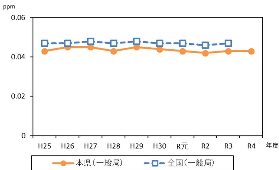
図2-4 本県及び全国の光化学オキシダント濃度の推移
