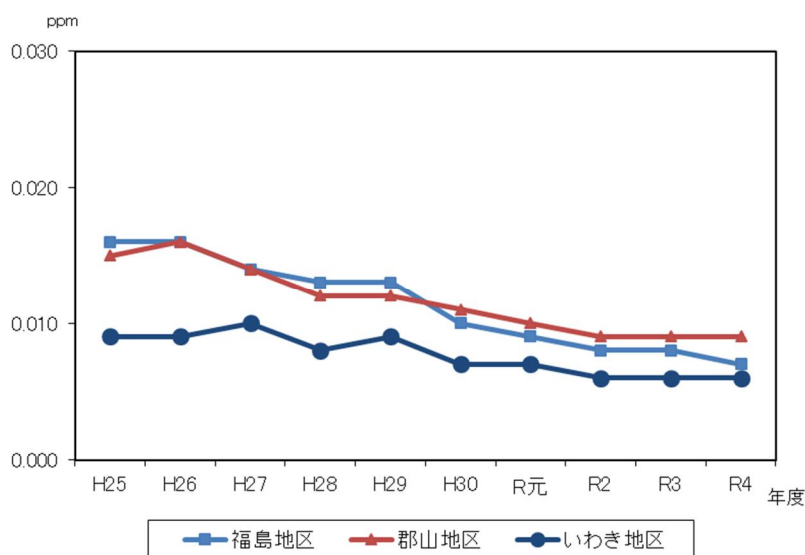
図 2-16 二酸化窒素（年平均値）の経年変化
