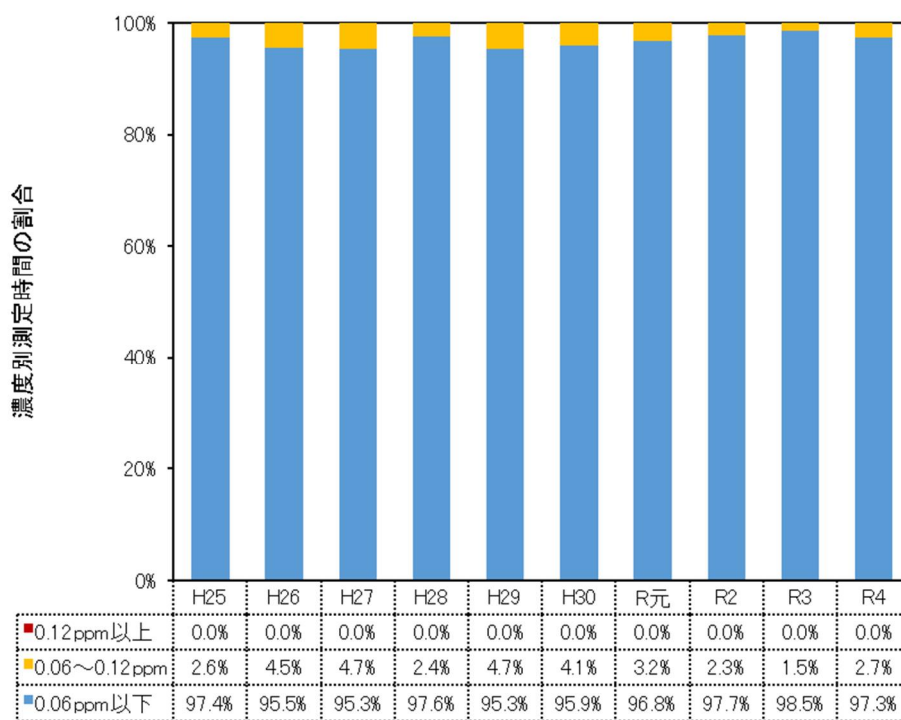
図 2-6 光化学オキシダント（昼間の1時間値）の濃度レベル別割合の推移
