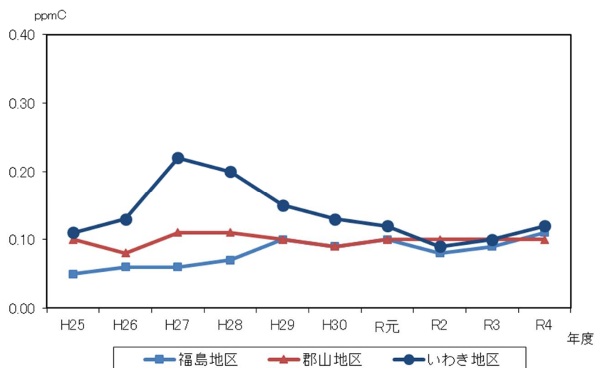
図 2-15 非メタン炭化水素（年平均値）の経年変化
