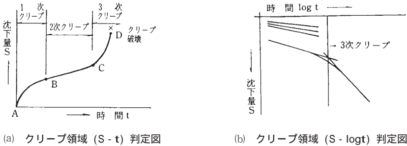
図5 - 1 天端沈下のクリープ領域判定図
