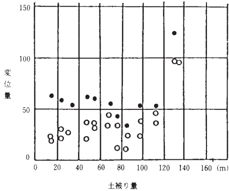
図5 - 3 内空変位量 - 土被り
