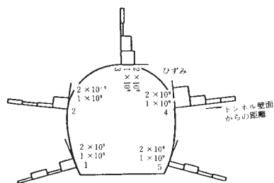
図6-2 地中ひずみ分布
