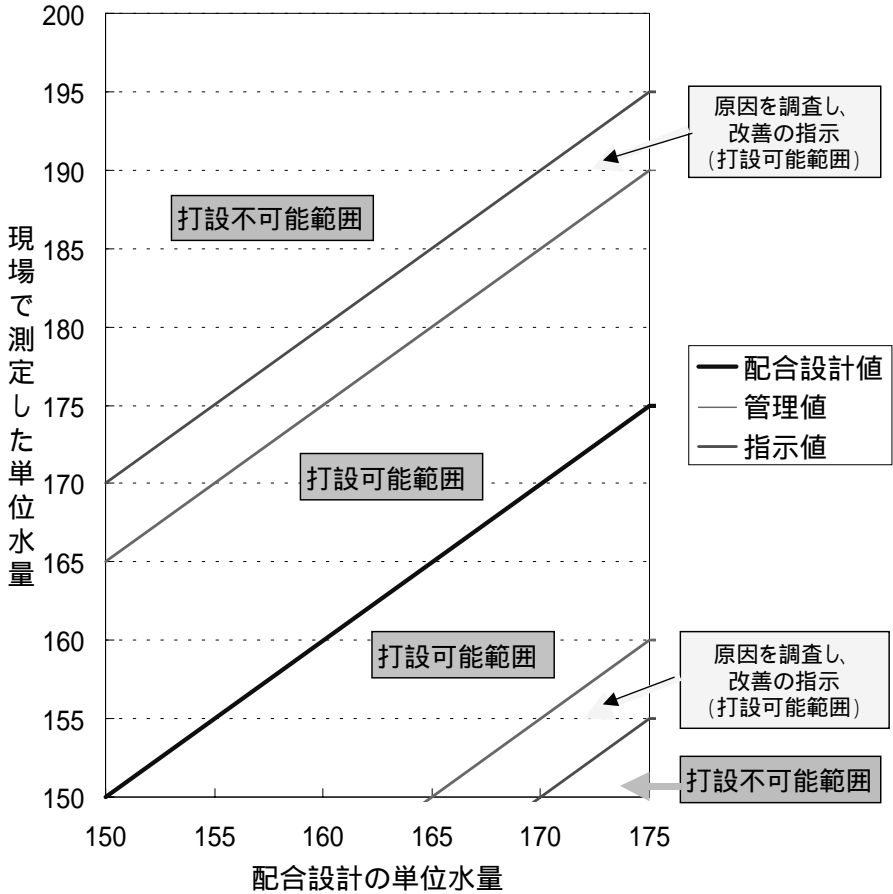
レディミクストコンクリートの 単位水量測定の管理図 (kg/m 3 )
