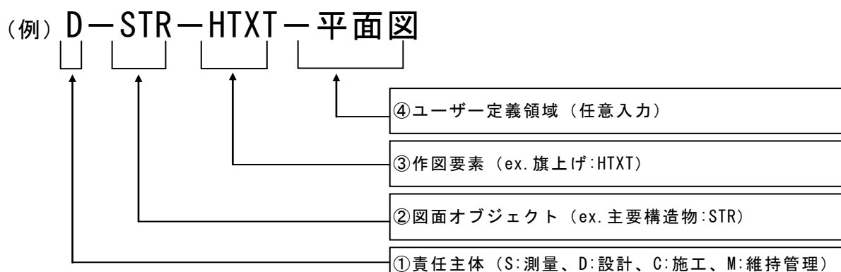
図 4-2 図面ファイルのレイヤ命名
