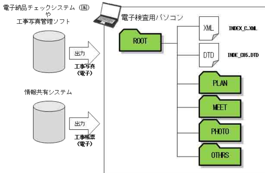
(b) 電子検査における工事写真、工事帳票の出力例
