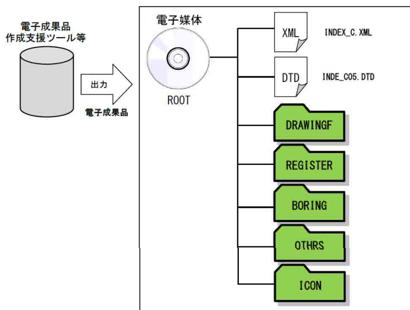
(a) 電子検査における電子成果品の出力例
