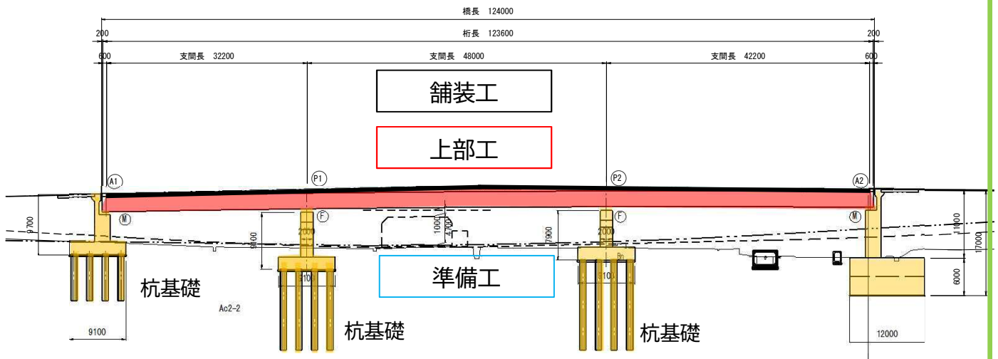
側面図
