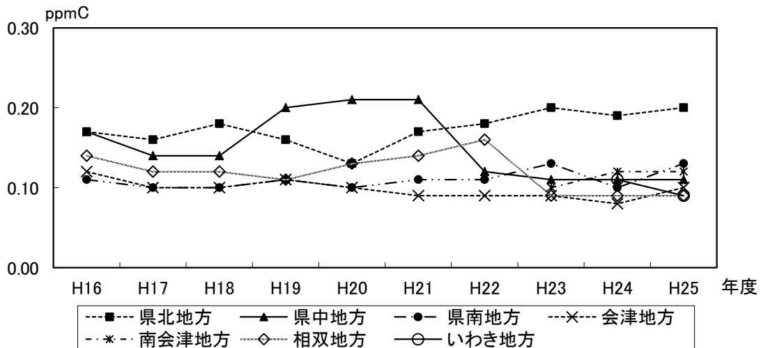
図-12 非メタン炭化水素(3時間平均値の年平均値)の経年変化
