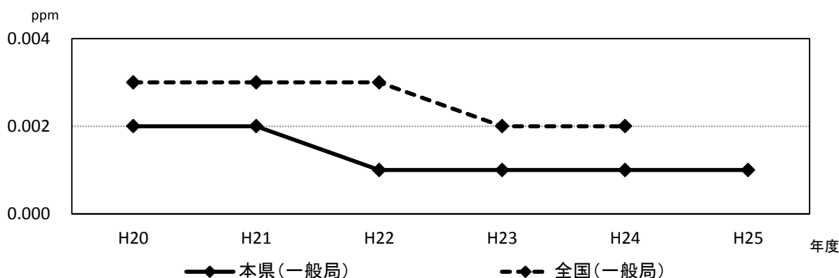
図-1 二酸化硫黄濃度の推移
