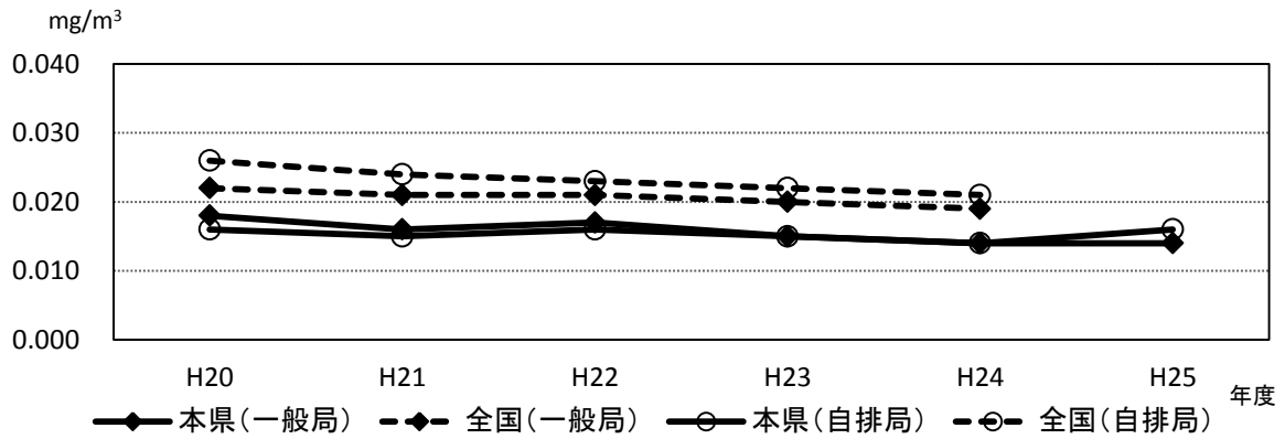
図-3 浮遊粒子状物質濃度の推移
