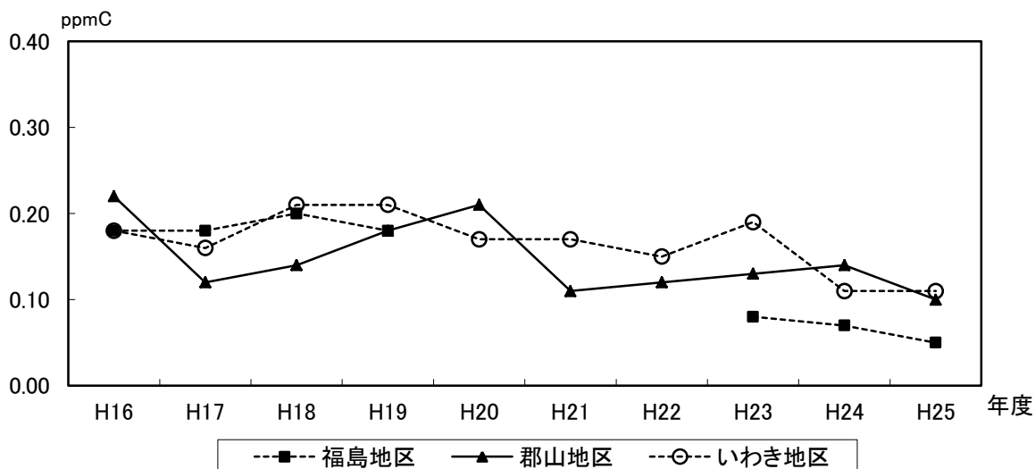
図-16 非メタン炭化水素(3時間平均値の年平均値)の経年変化
