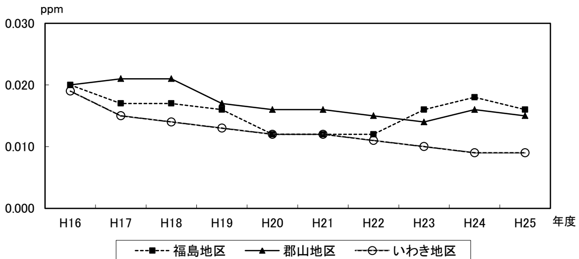
図-15 二酸化窒素濃度(年平均値)の経年変化
