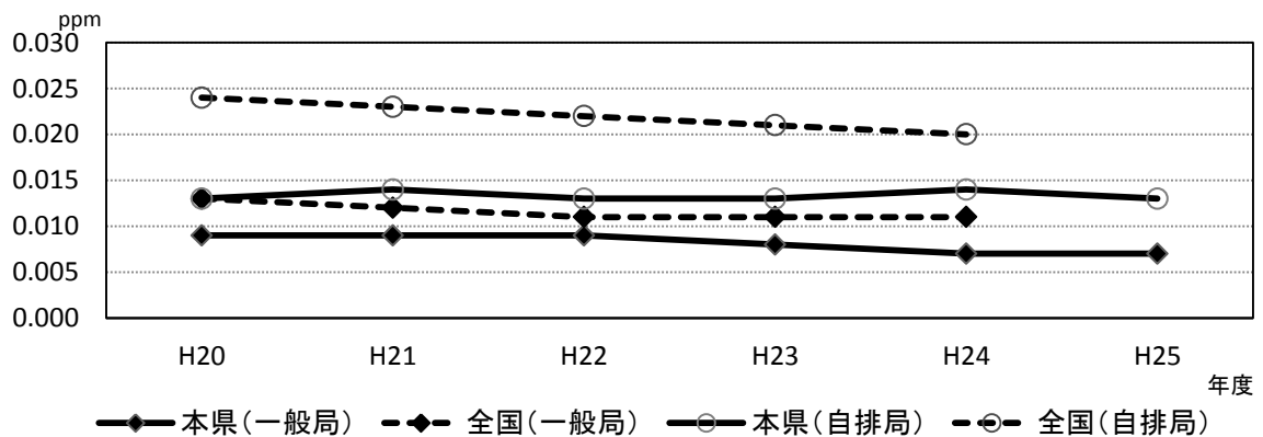
図-5 二酸化窒素濃度の推移
