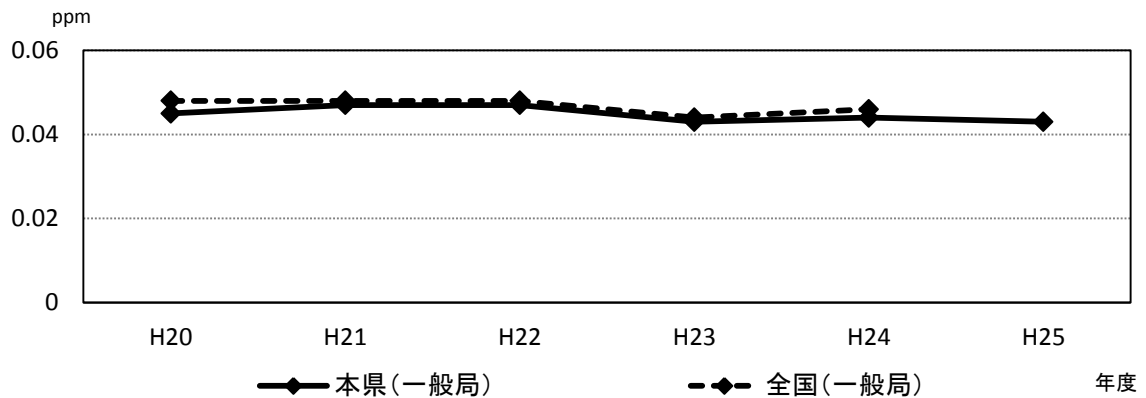
図-4 光化学オキシダント濃度の推移
