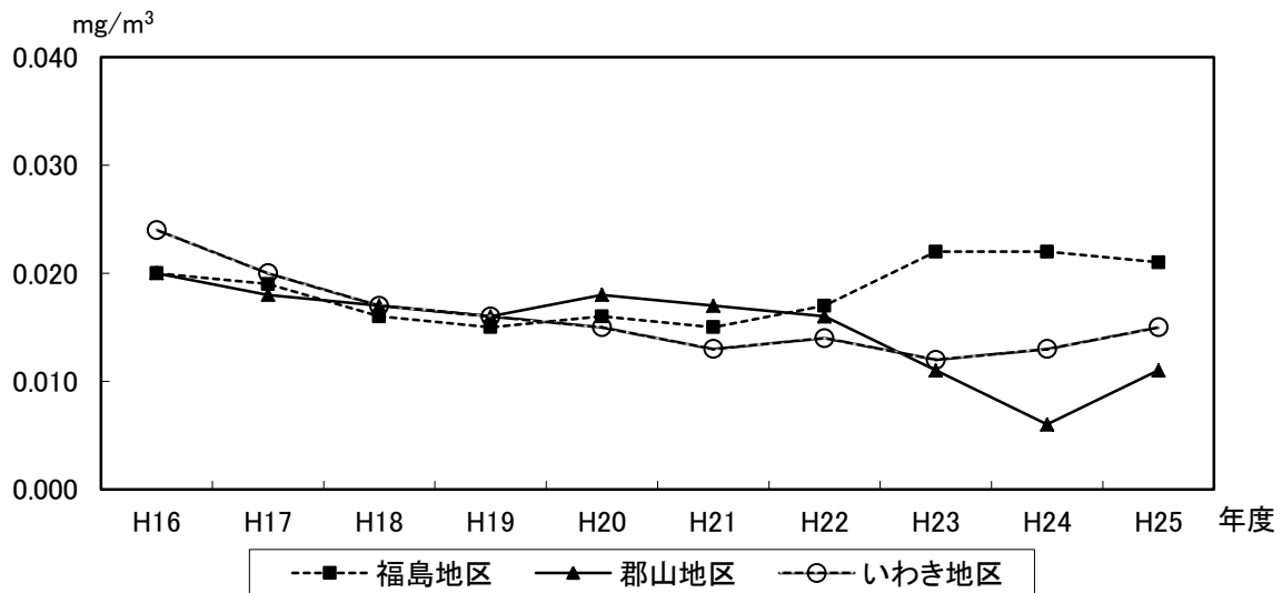
図-14 浮遊粒子状物質(年平均値)の経年変化
