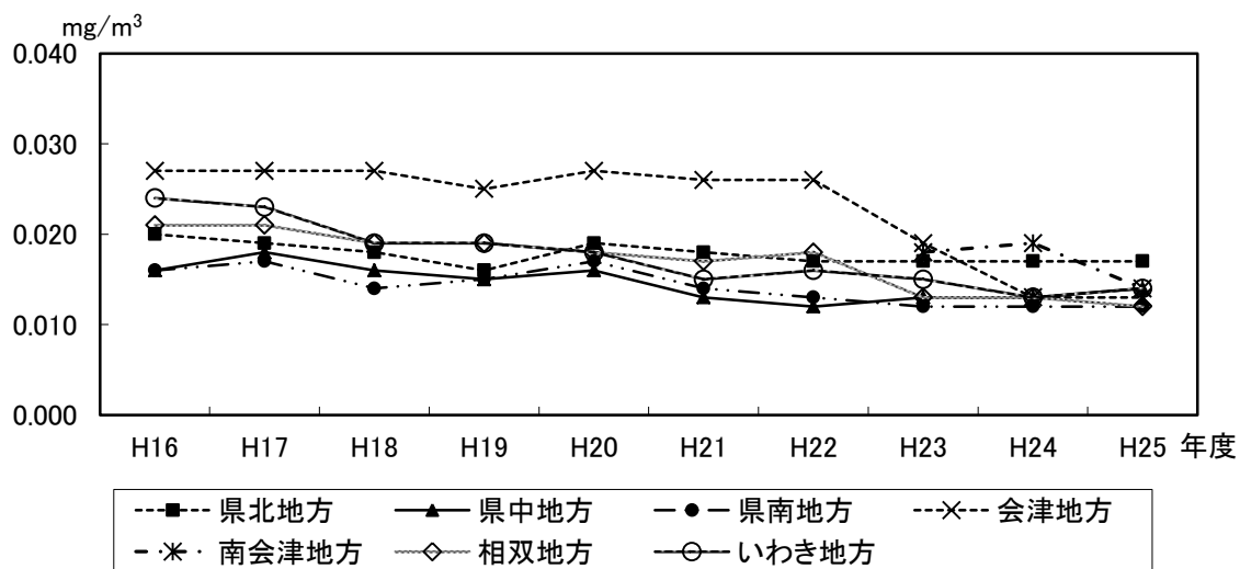
図-8 浮遊粒子状物質濃度(年平均値)の経年変化
