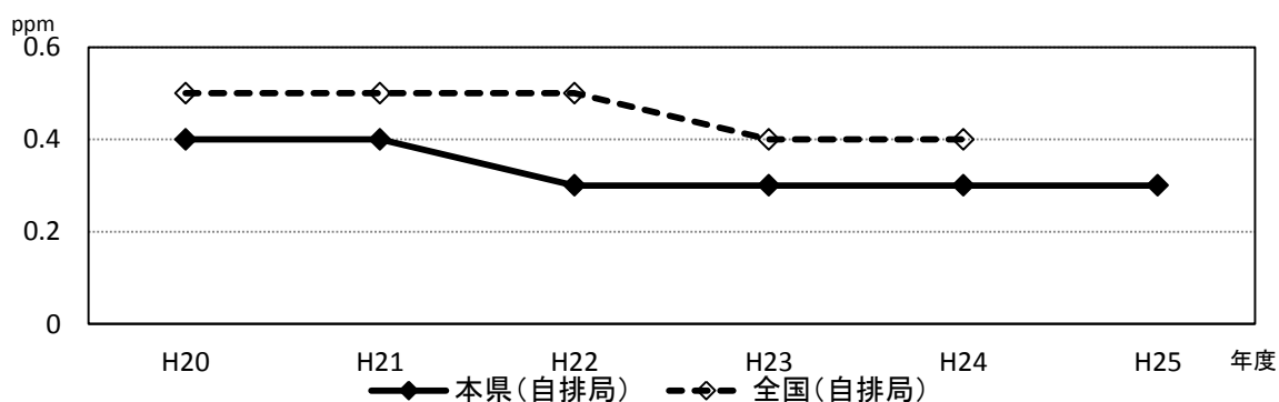
図-2 一酸化炭素濃度の推移
