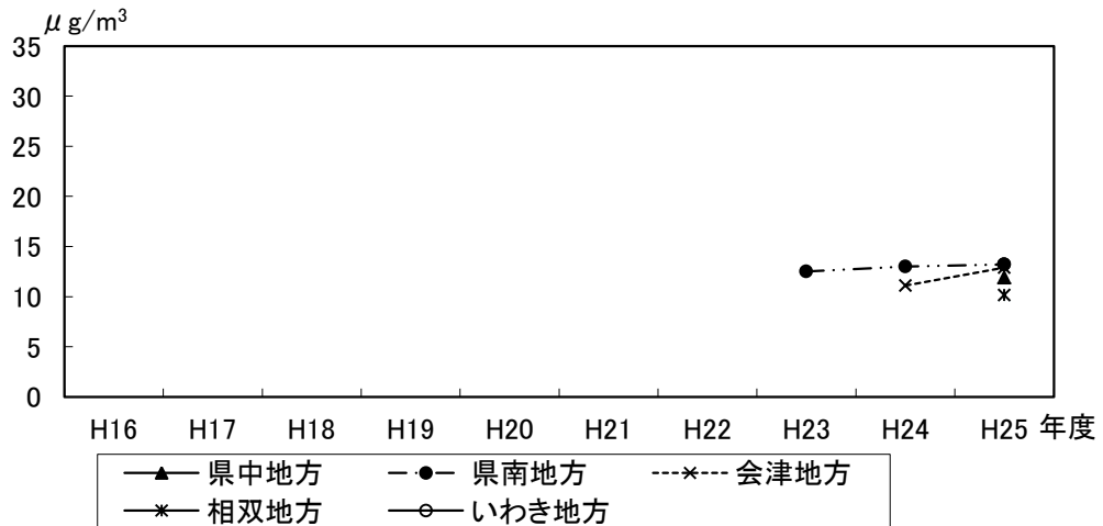
図-11 微小粒子状物質(年平均値)の経年変化
