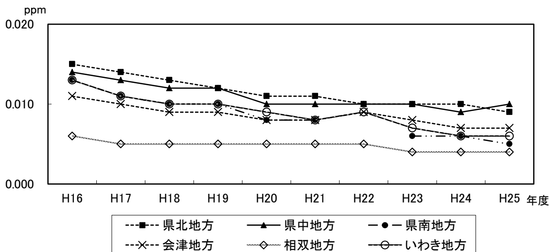
図-10 二酸化窒素濃度(年平均値)の経年変化
