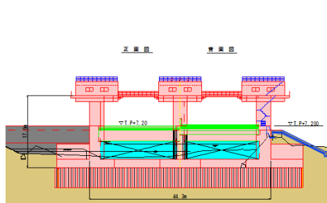
【正面図】
