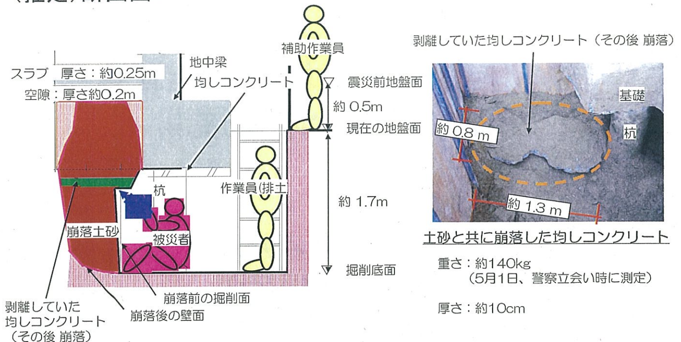
(推定)断面図1
