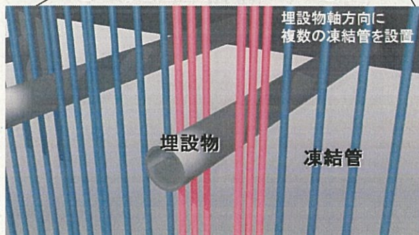
①凍結管建込み・ブライン循環
