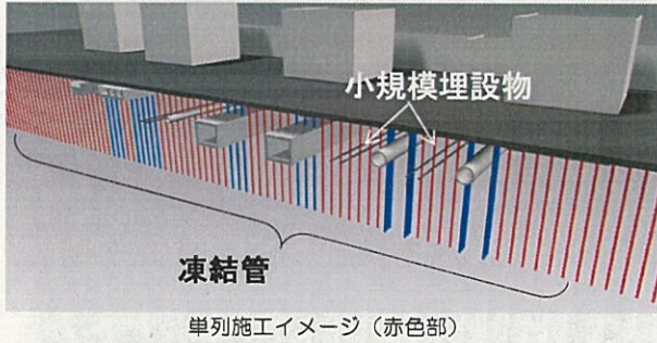
①凍結管建込み・ブライン循環
