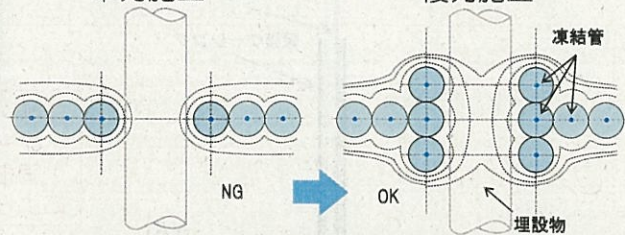
②凍土壁造成
