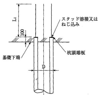
図 4.3.1 杭頭補強図 (1)
