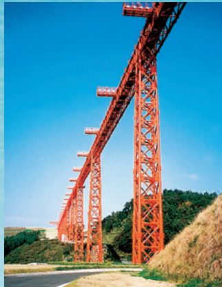
標準式進入灯 (PALS)
