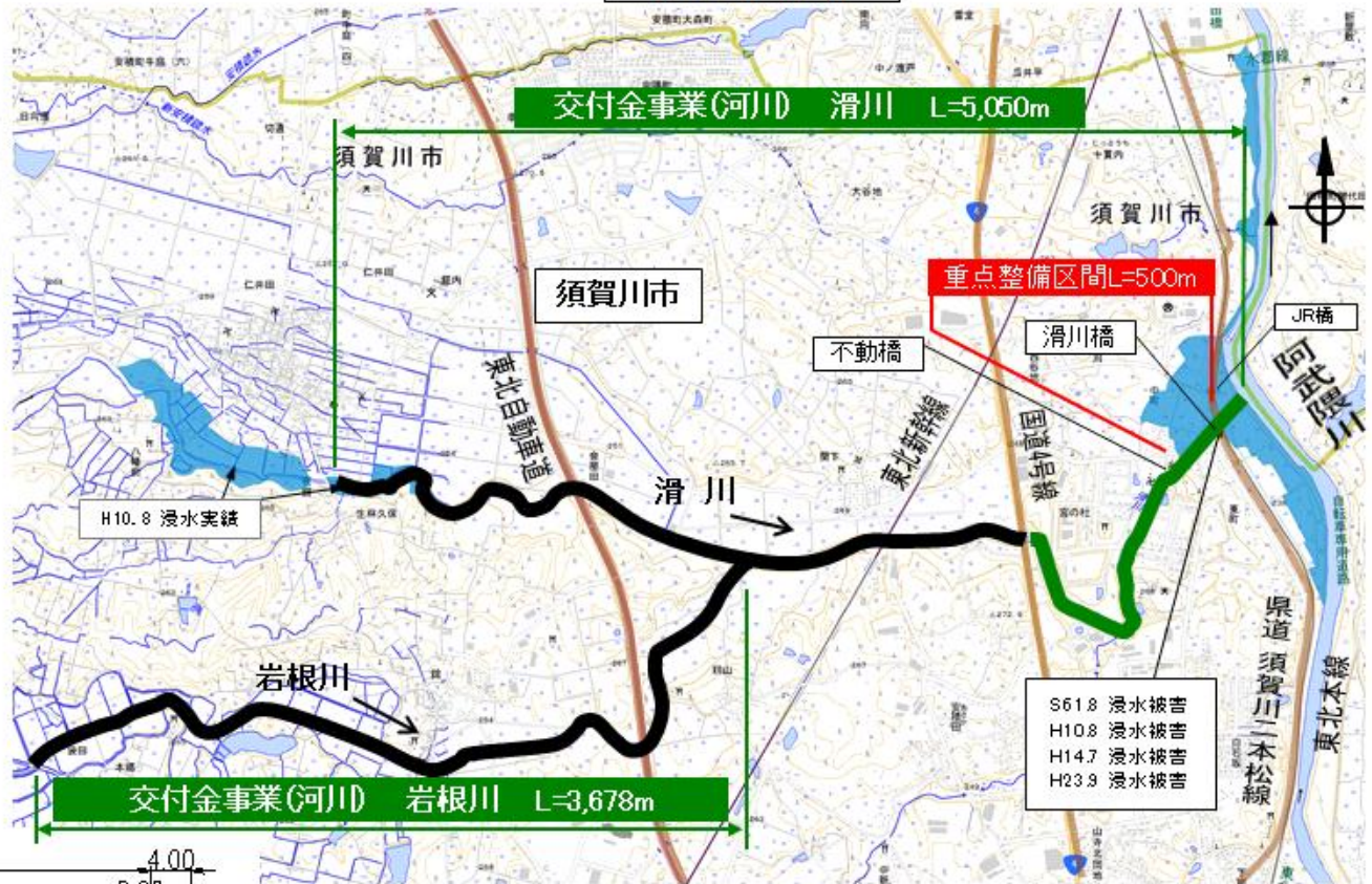
概略平面図
