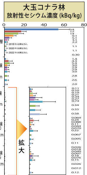
図3 土壌の深度別放射性セシウム濃度の変化
