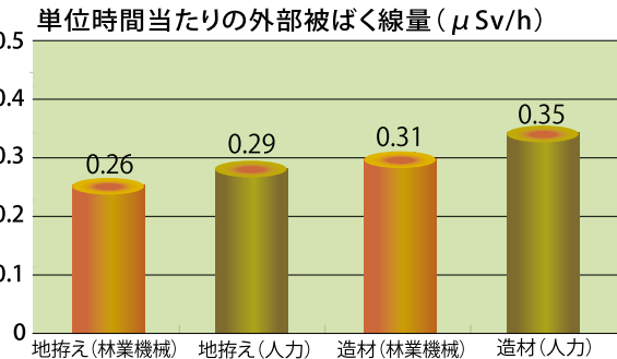
図 作業種ごとの単位時間当たり外部被ばく線量 資料：林野庁「平成26(2014)年度「森林における除染等実証事業」のうち「避難指示解除準備区域等における実証事業(田村市)」報告書」を基に作成
