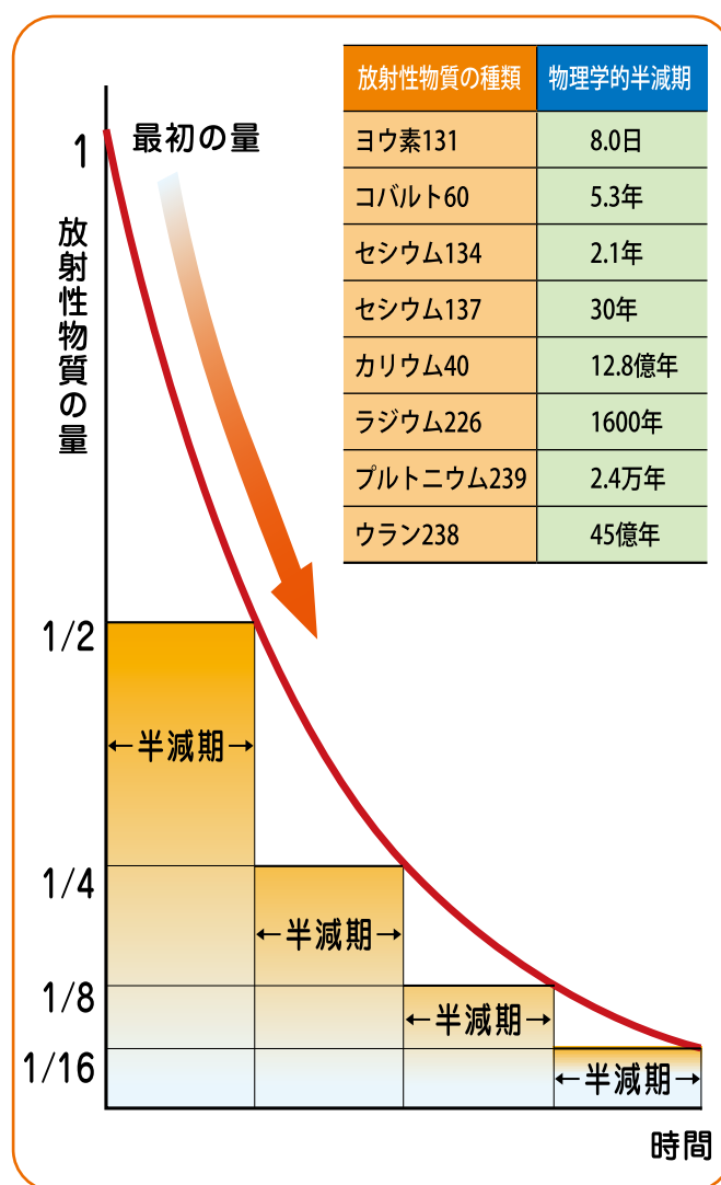
図 物理学的半減期
