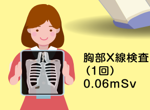
図 身の回りの放射線
