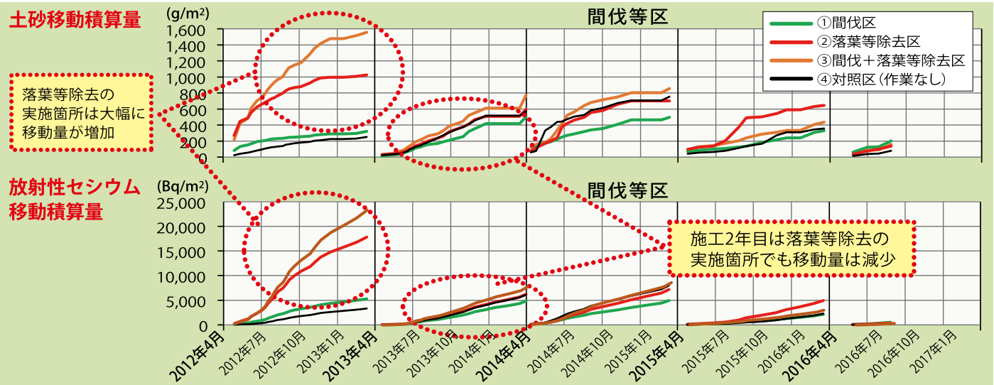
図 森林施業等実施後の土砂等及び放射性セシウムの移動積算量の推移(間伐) 資料：林野庁「森林における放射性物質対策技術検証・開発事業の成果」(2017年度)を基に作成
