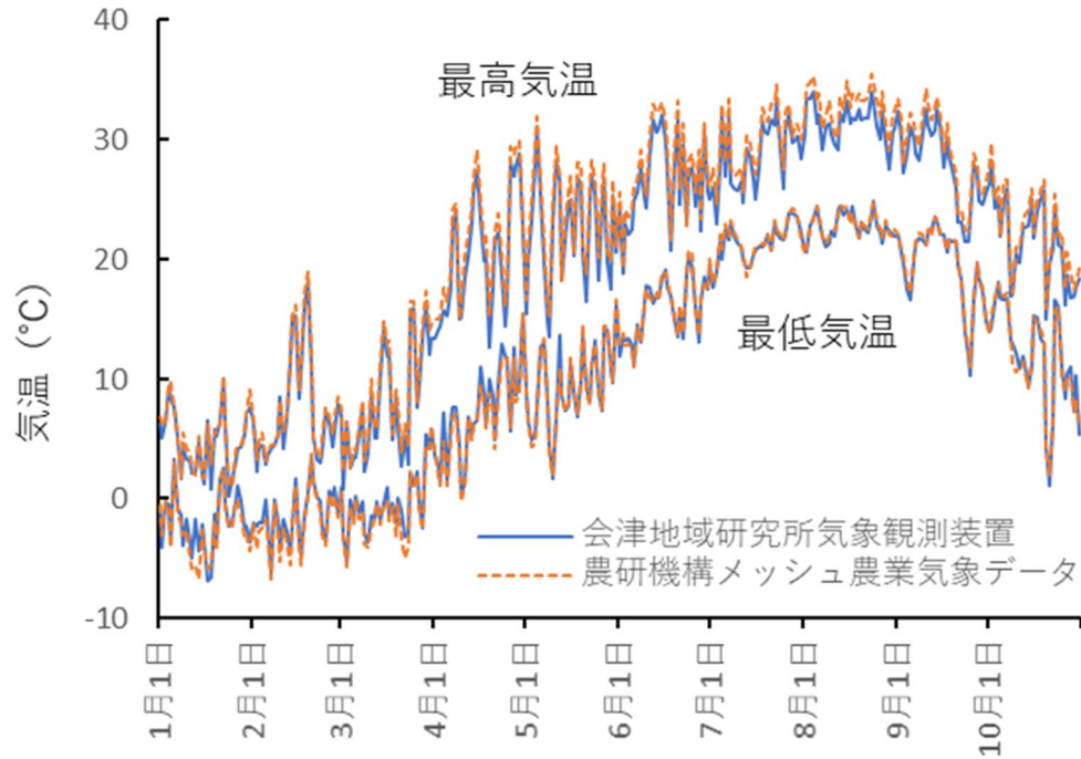
図1 農研機構メッシュ農業気象データと実測値の比較（2024 年）
