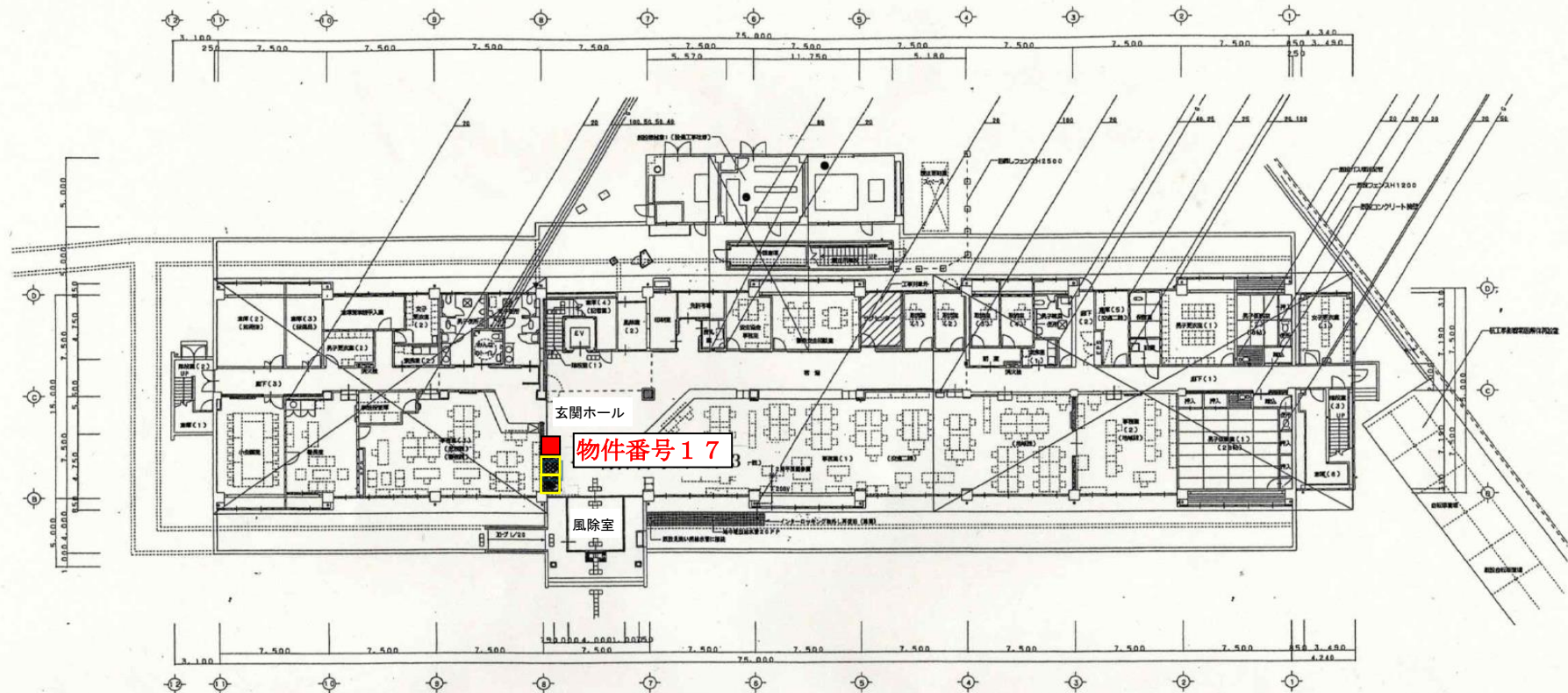
いわき中央警察署 本庁舎1階配置図
