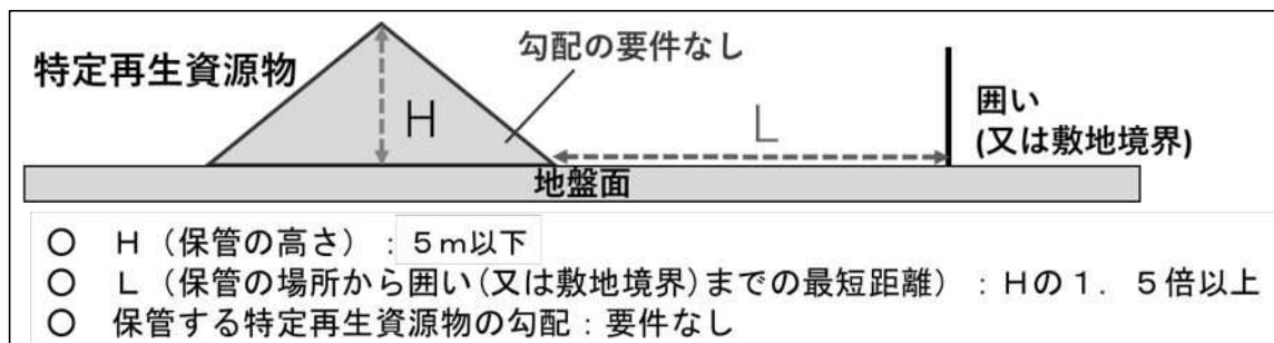
図5-1 保管高さの図示（勾配要件なし）
