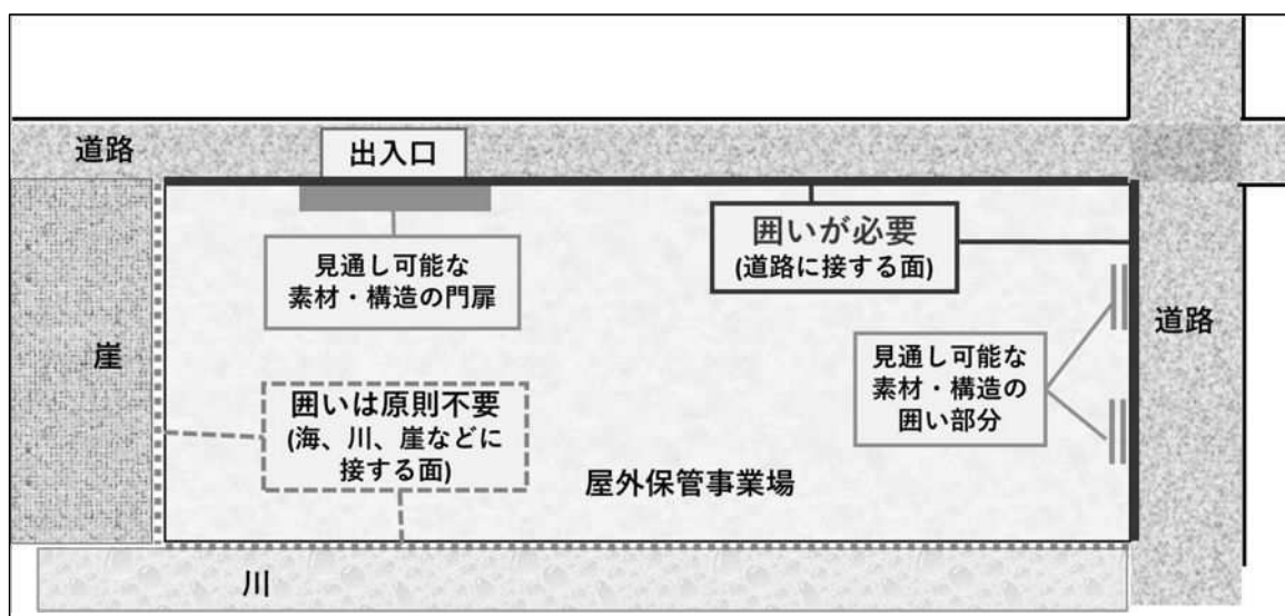
図3 囲いの構造の例（平面図）
