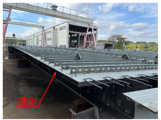
製作中の橋桁 (R7.10.29撮影)
