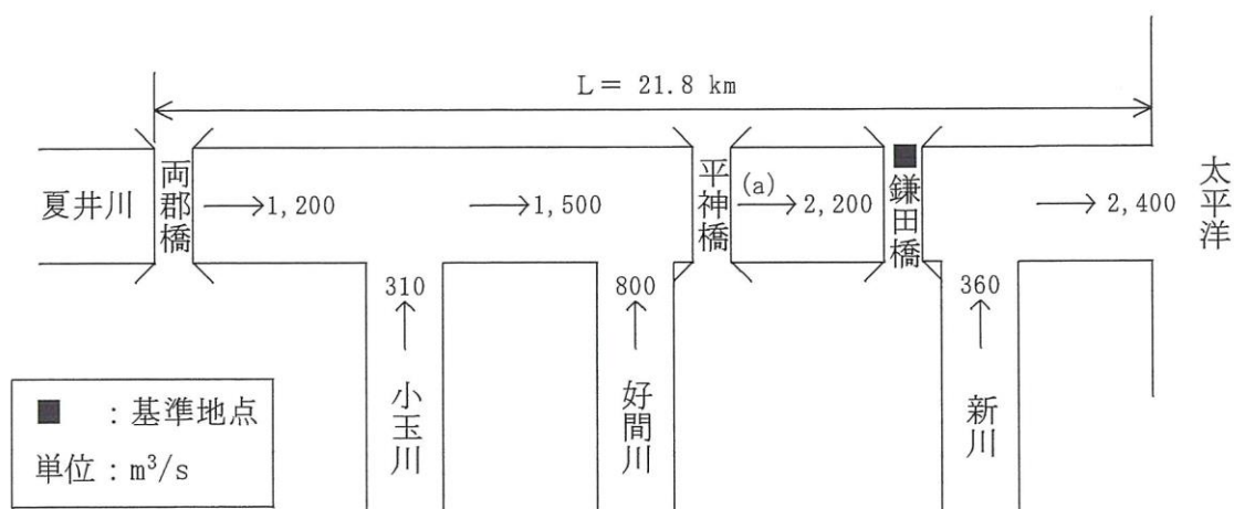
流量配分図
