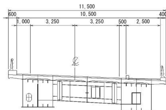
橋梁部 (ひばら橋 L=43.0m)
