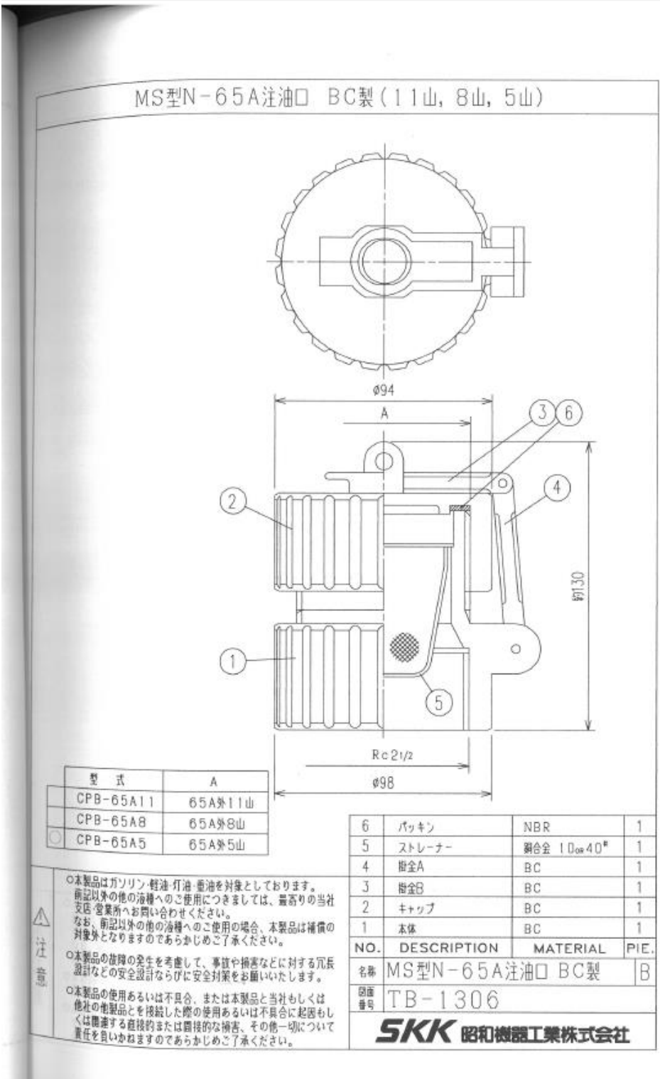
白河高等学校給油口(図面)
