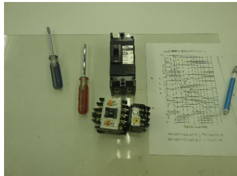
実習の様子① (ブレーカー分解実習)
