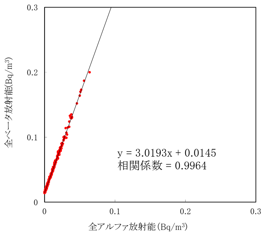
大気浮遊じんの全アルファ・全ベータ放射能の相関図 (MP-7) (令和7年4月～令和7年6月)
