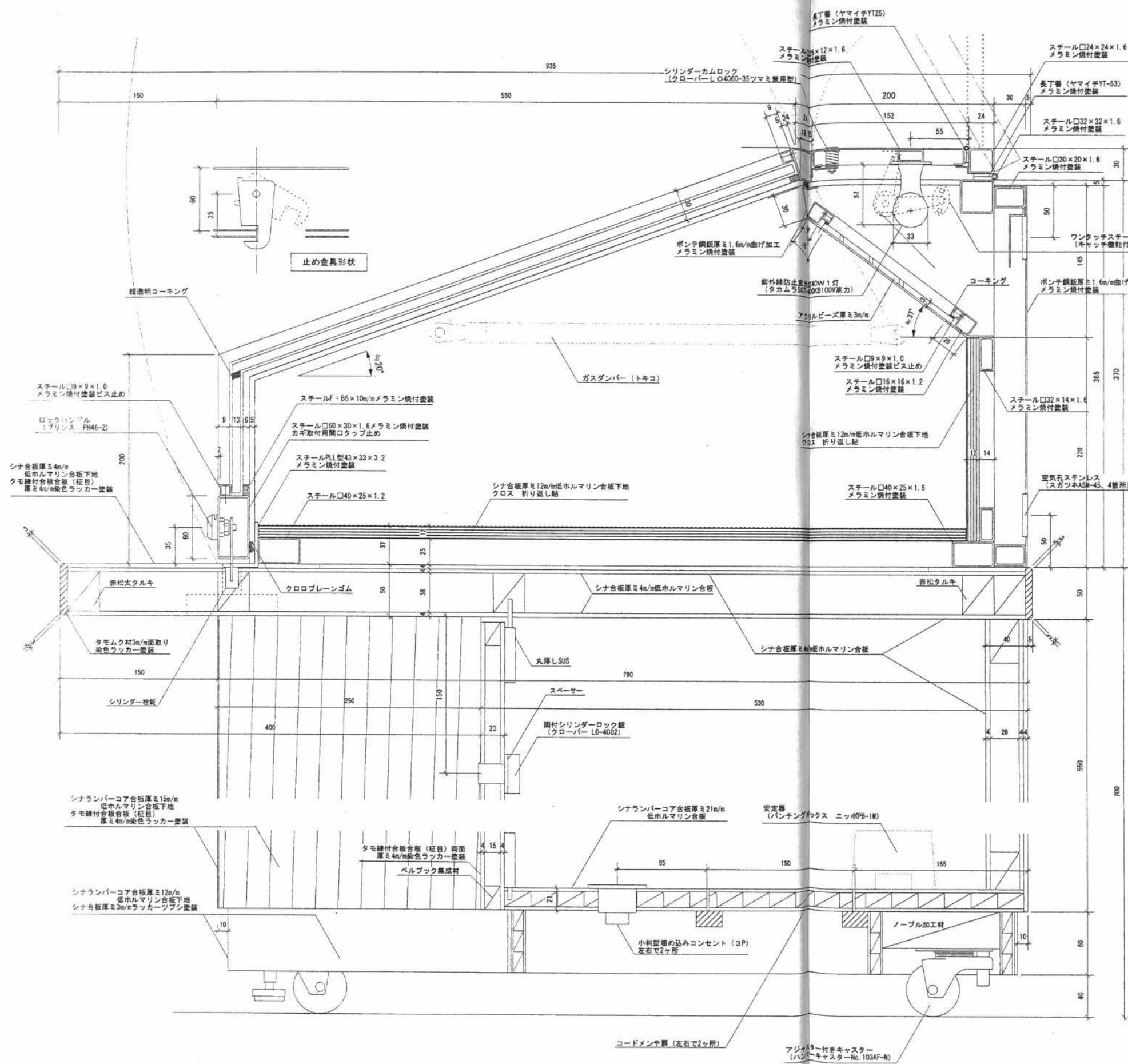
縱斷面詳細圖
