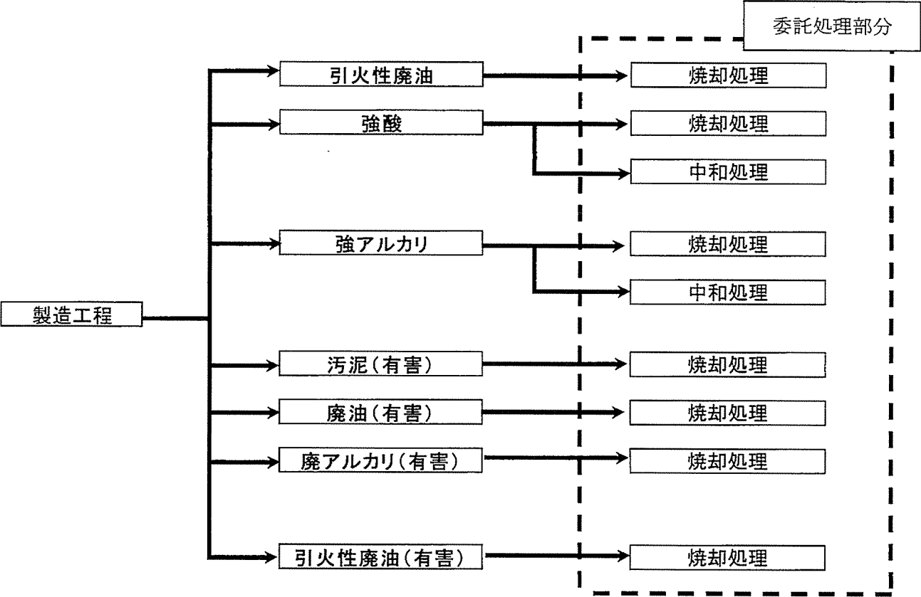
別紙 1 特別管理産業廃棄物の一連の処理の工程
