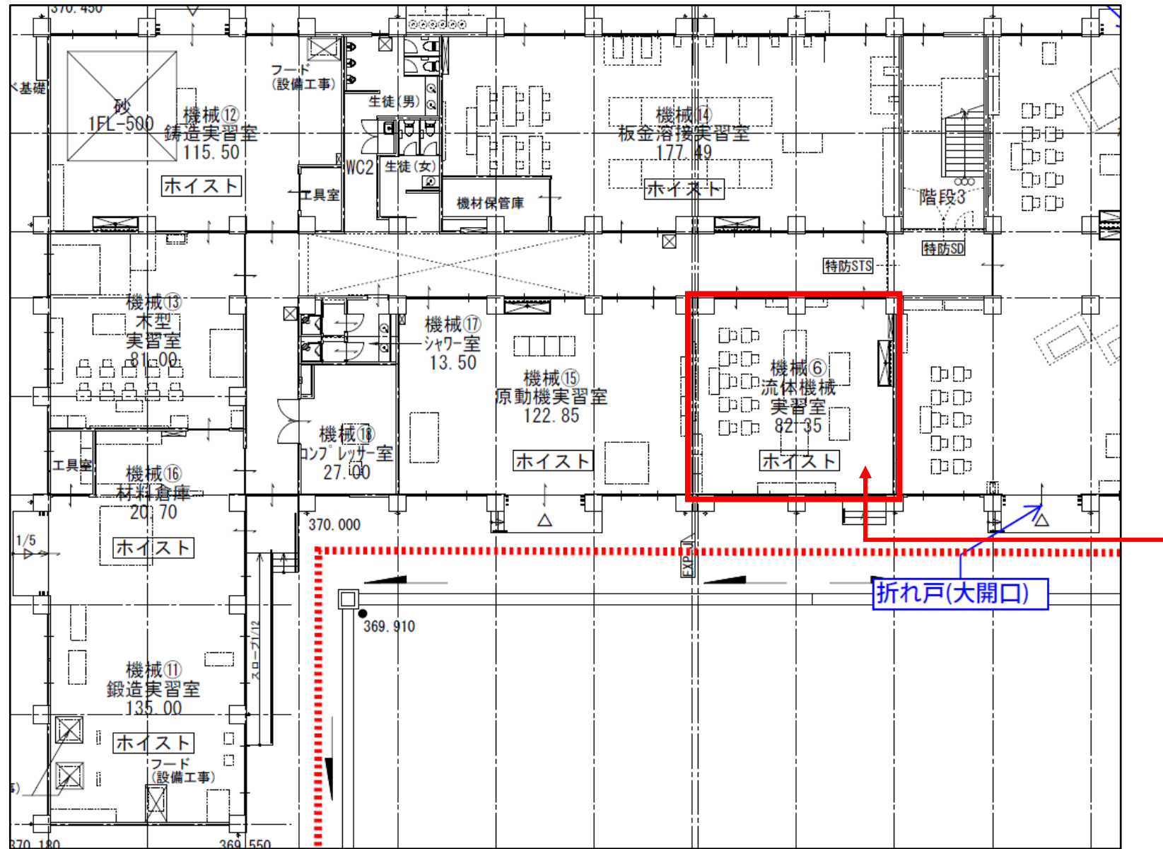
福島県立白河実業高等学校 実習棟平面図
