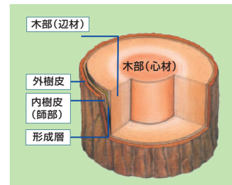
図2 樹幹の構造
