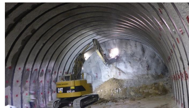
国道114号 川俣町工区関場トンネル 令和4年3月2日 貫通
