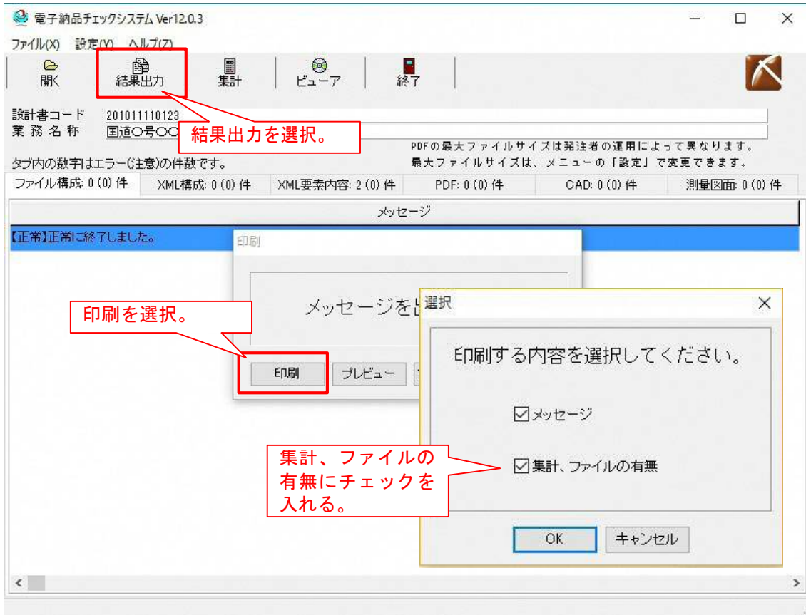
図 6-18 チェック結果の印刷内容の選択画面
