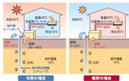
安定した地中温度を利用するメリット 注）図中の温度はイメージです。
