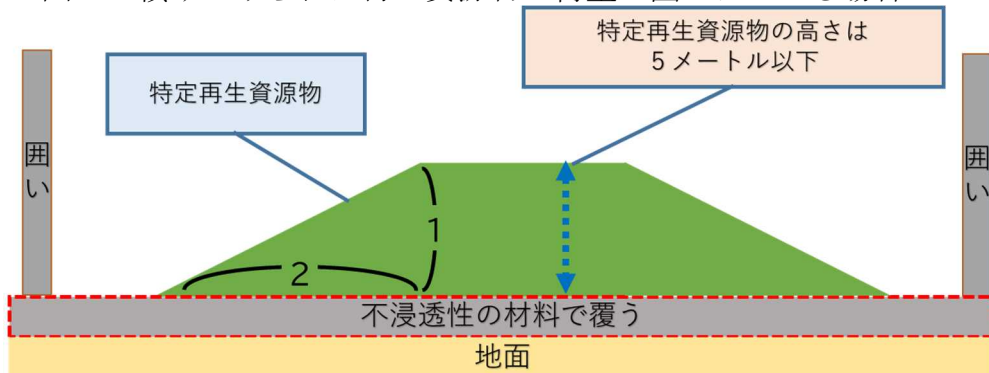
図2 積み上げられた再生資源物の荷重が囲いにかからない場合
