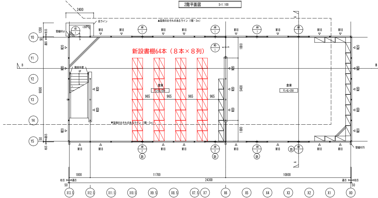
1階平面図 S=1:100
