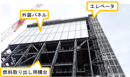
(写真1-2) 2号機燃料取り出し用構台の状況② (南側から撮影)
