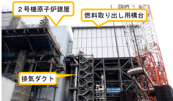
(写真2-1) 2号機換気設備排気ダクトの設置状況① (西側から撮影)
