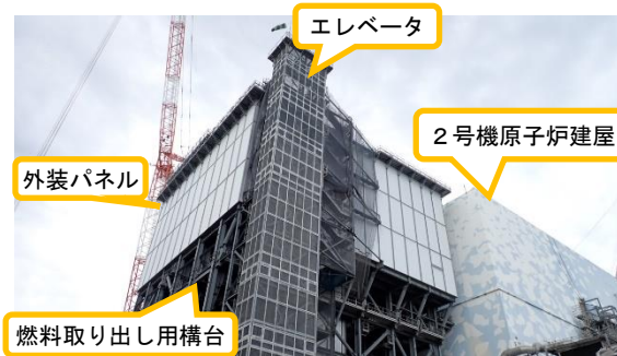
(写真1-3) 2号機燃料取り出し用構台の状況③ (東南側から撮影)
