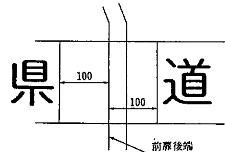
図-3 ドア付近文字の表示方法詳細
