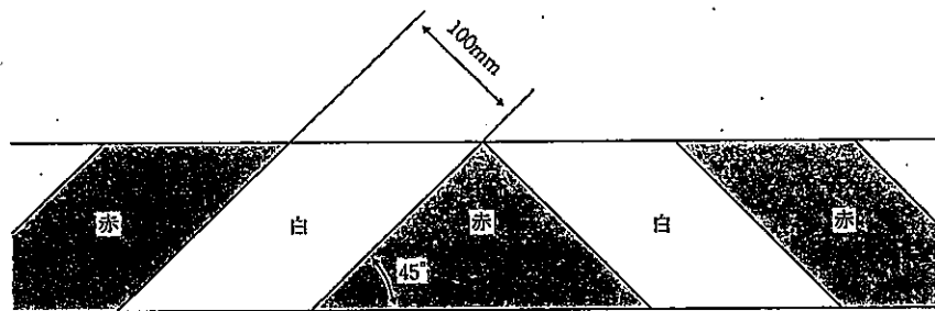
車両前後部の赤白縞
