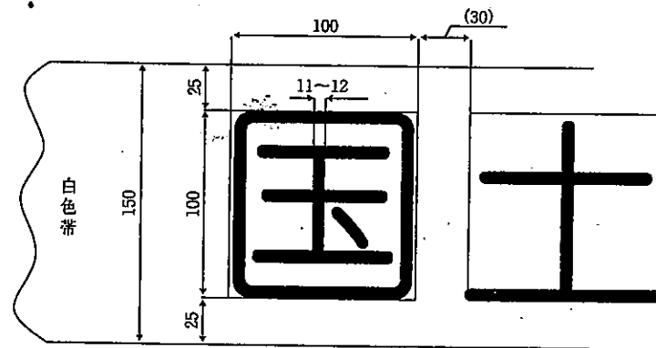
図-4 文字の形式および寸法
