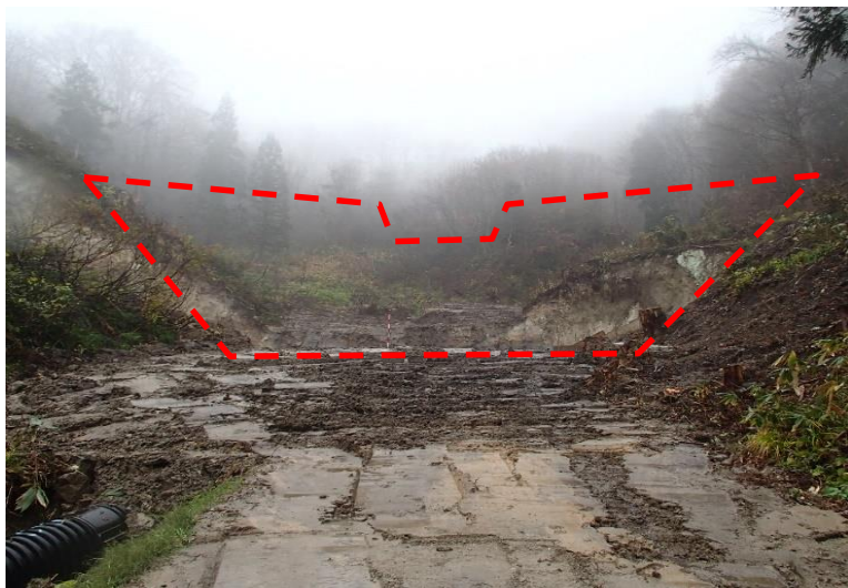
にしたづらさわ 西田面沢（会津若松市）砂防堰堤工
