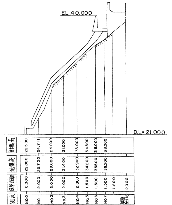
余水路縦断面図 縮尺 1/200
