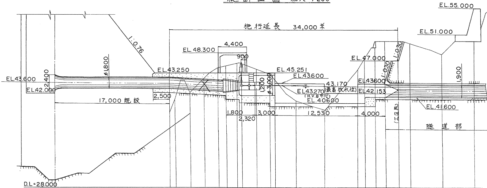
縦断面図 縮尺 1/200
