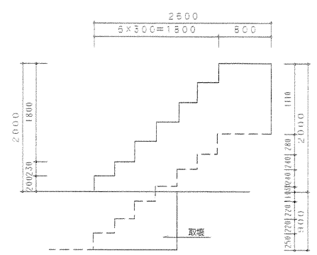
B-B断面
