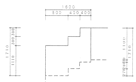
A-A断面
