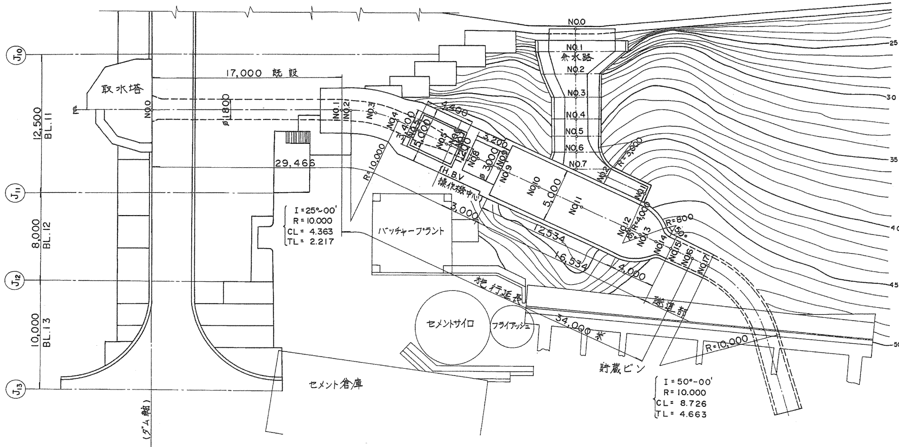
平面図 縮尺 1/200
