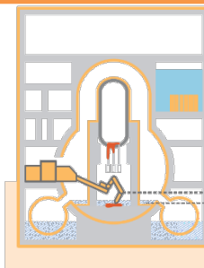
ロボットが燃料デブリと思われる堆積物の持ち上げに成功(2号機:2019年2月)
