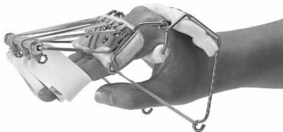
↑ MP屈曲装具（ナックルバンダー）指伸展補助付
