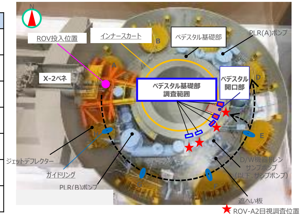
原子炉格納容器地下階模型
