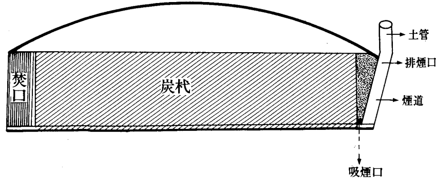
3-4図 炭窯の断面図
