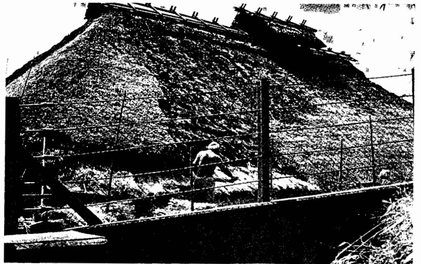
2-28 萱の屋根葺き 戦前、戦後の萱葺きは、屋根の大きさにより多くの萱手職人や手伝いの人があったが、現在は萱屋根葺きの光景が、ほとんど見られなくなった。
