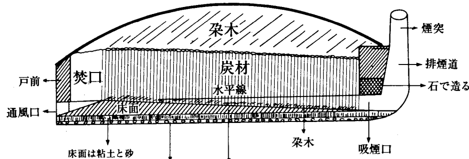
3-3図 窯の平面図
