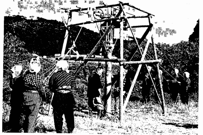
2-32 土突き 土突き棒で土をついて固める。土突き棒は生の松の木を使い長さ一丈(3m)、太さは元の方が直径七寸五分(23cm)くらい。先端には鉄の輪がはめてある。
