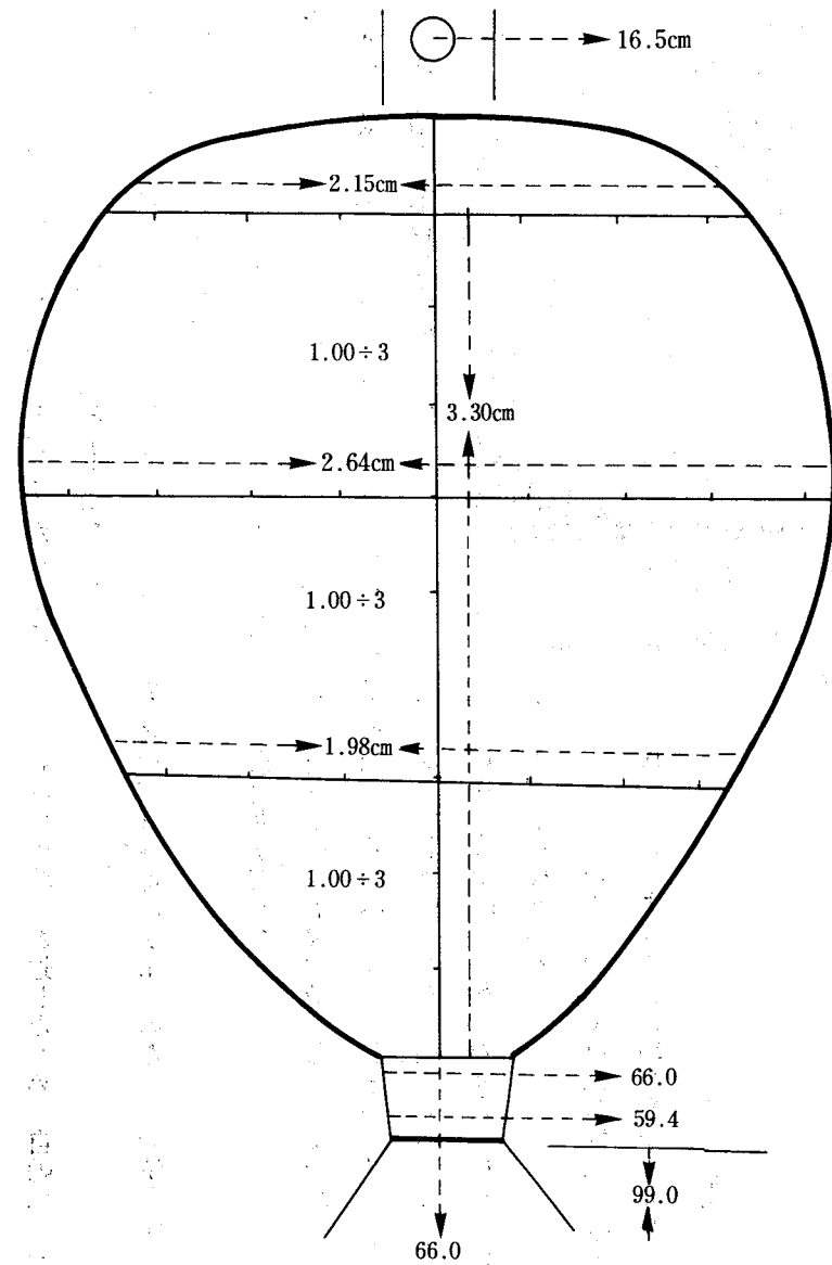
3-1図 炭窯の地割平面図
