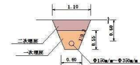
標準断面図 (小排水路)
