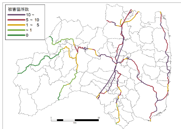
▲想定東北地方太平洋沖地震による鉄道の路線の被害箇所数
