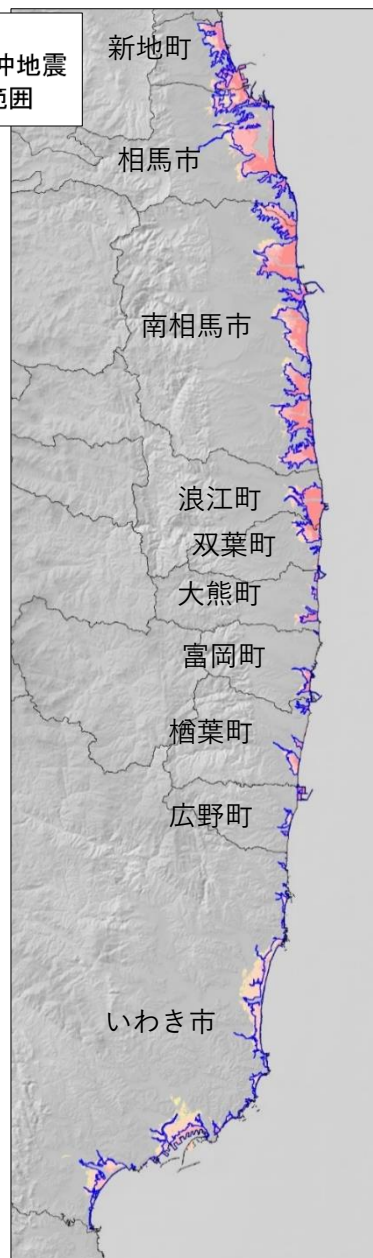
▲想定東北地方太平洋沖地震で想定される浸水深分布
