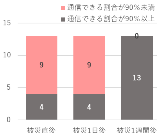
▲想定東北地方太平洋沖地震の地震が発生した場合の時間の経過別・不通回線率別の浜通り地方の市町村数
