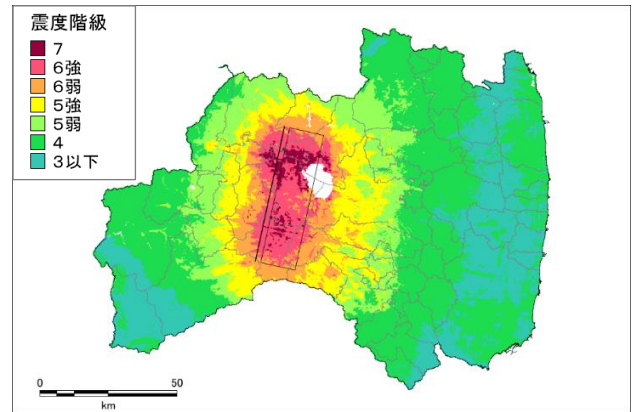
▲会津盆地東縁断層帯の地震の震度分布
