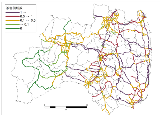
▲想定東北地方太平洋沖地震による緊急輸送道路の被害率分布図
