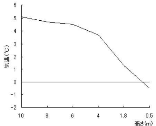
図5 逆転層の出現状況(小松1994)
