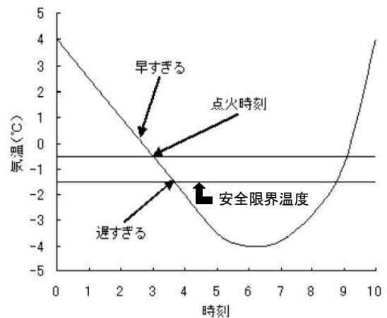
図4 危険限界温度と点火時刻
