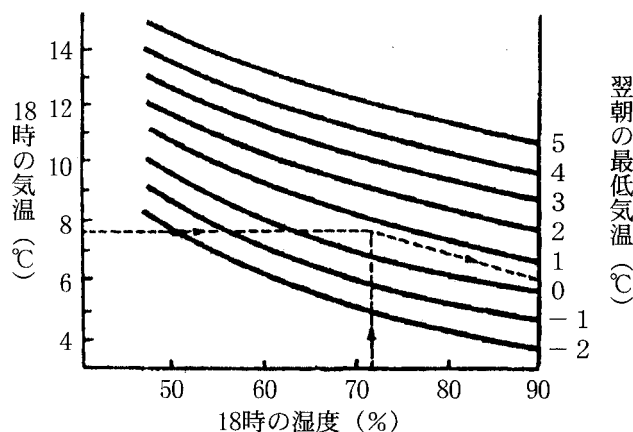
図3 18時の気温、湿度から翌朝の最低気温を推定する図（名古屋地方気象台）
