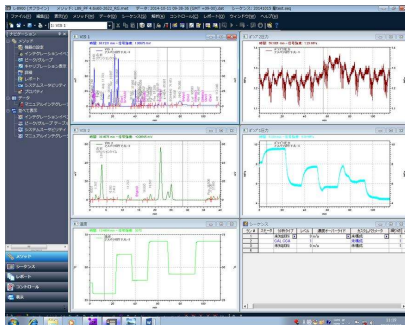
測定画面
