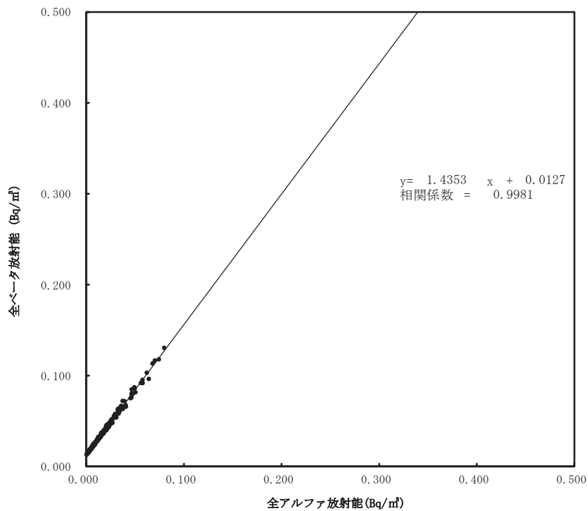
大気浮遊じんの全アルファ・全ベータ放射能の相関図 (6時間連続集じん・6時間放置後) (令和4年7月～9月) (南相馬市泉沢)
