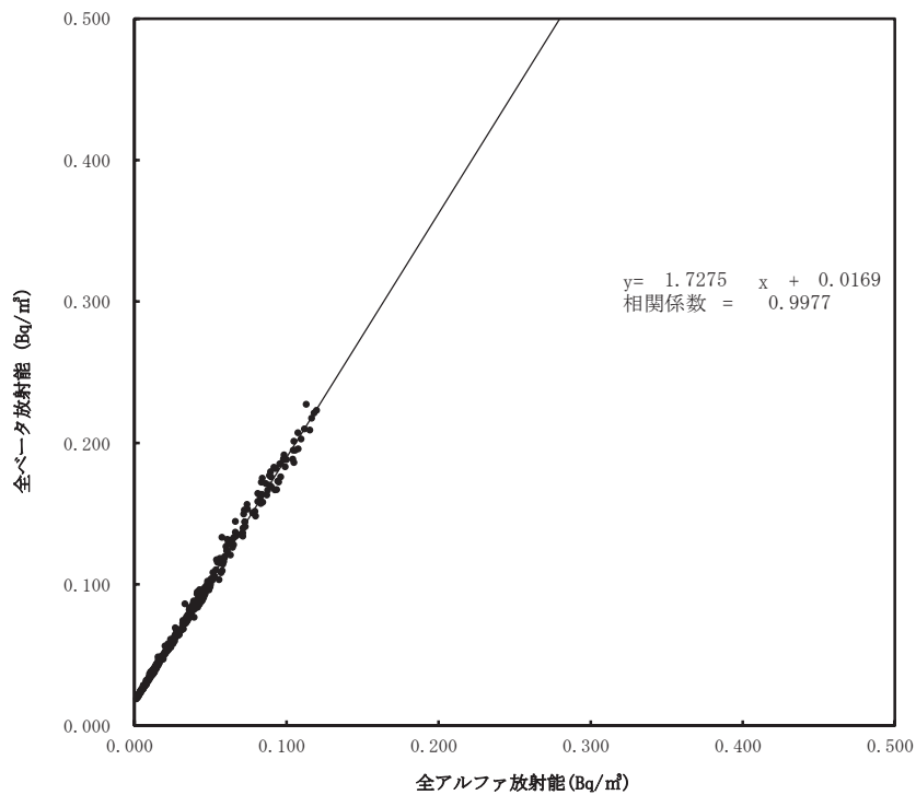
大気浮遊じんの全アルファ・全ベータ放射能の相関図 (6時間連続集じん・6時間放置後) (令和4年7月～9月) (浪江町大柿ダム)
