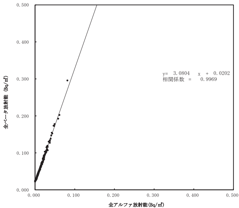
大気浮遊じんの全アルファ・全ベータ放射能の相関図 (6時間連続集じん・6時間放置後) (令和4年7月～9月) (飯館村伊丹沢)
