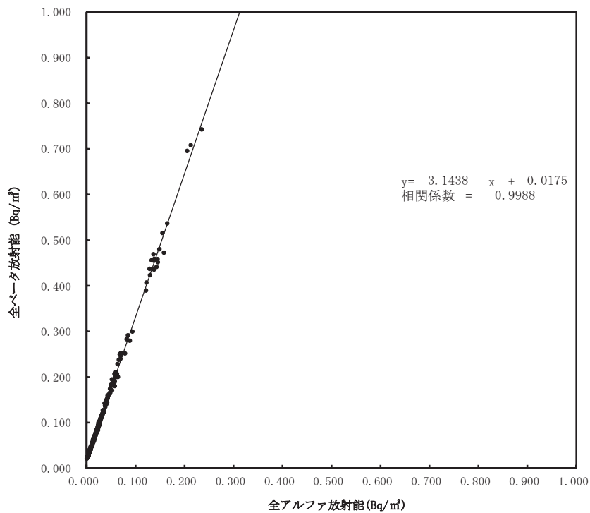
大気浮遊じんの全アルファ・全ベータ放射能の相関図 (6時間連続集じん・6時間放置後) (令和4年7月～9月) (大熊町大野)
