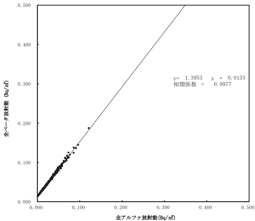
大気浮遊じんの全アルファ・全ベータ放射能の相関図 (6時間連続集じん・6時間放置後) (令和4年7月～9月) (檜葉町木戸ダム)
