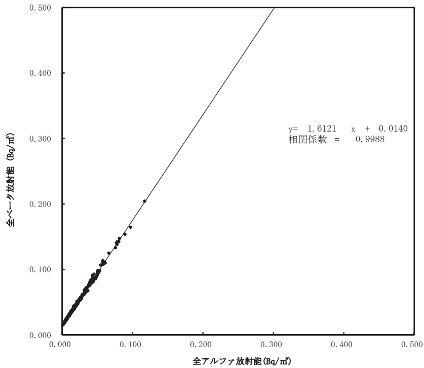
大気浮遊じんの全アルファ・全ベータ放射能の相関図 (6時間連続集じん・6時間放置後) (令和4年7月～9月) (広野町小滝平)
