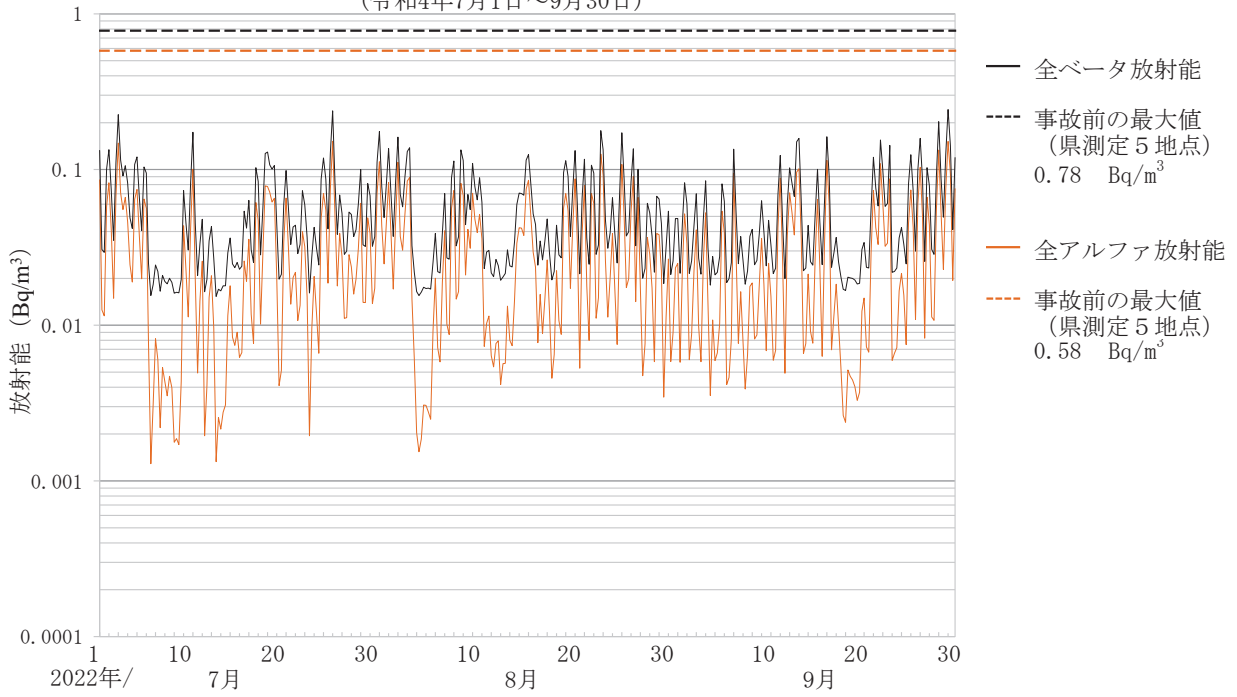
大気浮遊じんの全アルファ及び全ベータ放射能の推移 (6時間連続集じん・6時間放置後測定) 7 川内村下川内 (令和4年7月1日～9月30日)
