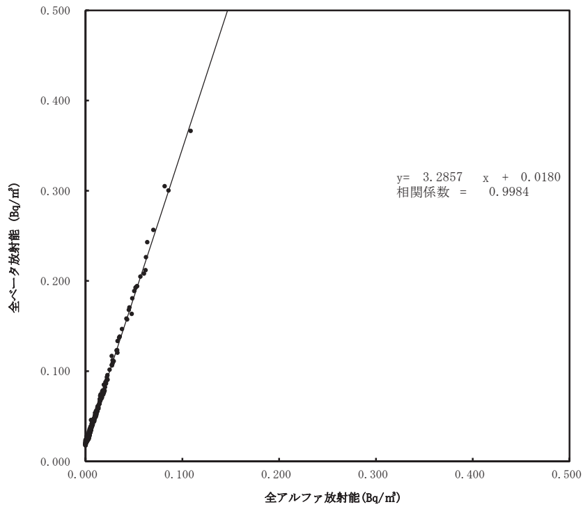
大気浮遊じんの全アルファ・全ベータ放射能の相関図 (6時間連続集じん・6時間放置後) (令和4年7月～9月) (大熊町大沢)
