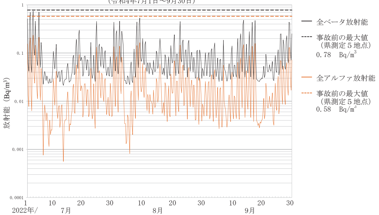
大気浮遊じんの全アルファ及び全ベータ放射能の推移 (6時間連続集じん・6時間放置後測定) 8 大熊町大野 (令和4年7月1日～9月30日)
