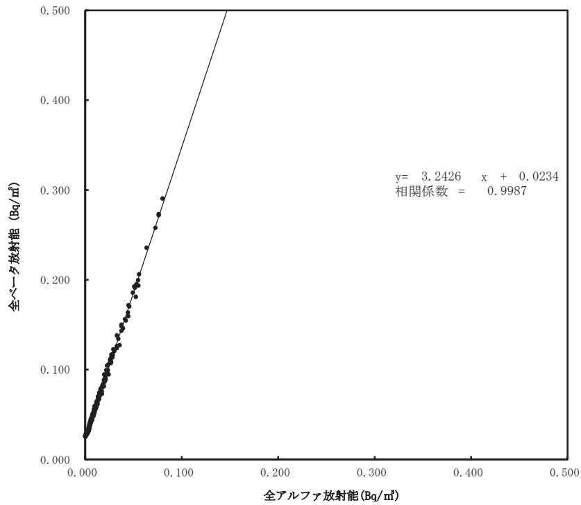
大気浮遊じんの全アルファ・全ベータ放射能の相関図 (6時間連続集じん・6時間放置後) (令和4年7月～9月) (南相馬市萱浜)
