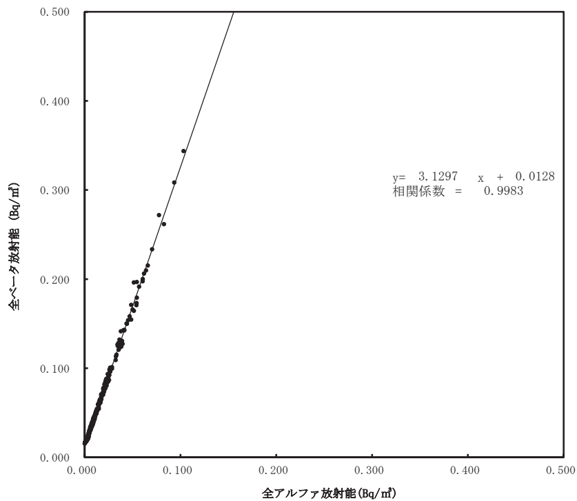
大気浮遊じんの全アルファ・全ベータ放射能の相関図 (6時間連続集じん・6時間放置後) (令和4年7月～9月) (富岡町富岡)
