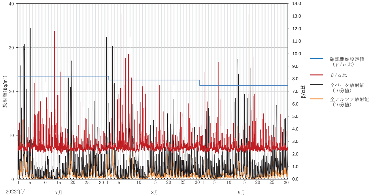
大気浮遊じんの全アルファ及び全ベータ放射能の推移（集じん中測定） 21 大熊町向畑 （令和4年7月1日～9月30日）
