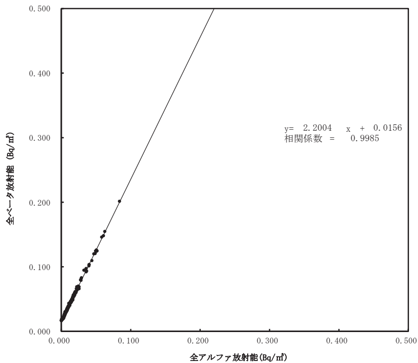
大気浮遊じんの全アルファ・全ベータ放射能の相関図 (6時間連続集じん・6時間放置後) (令和4年7月～9月) (双葉町郡山)
