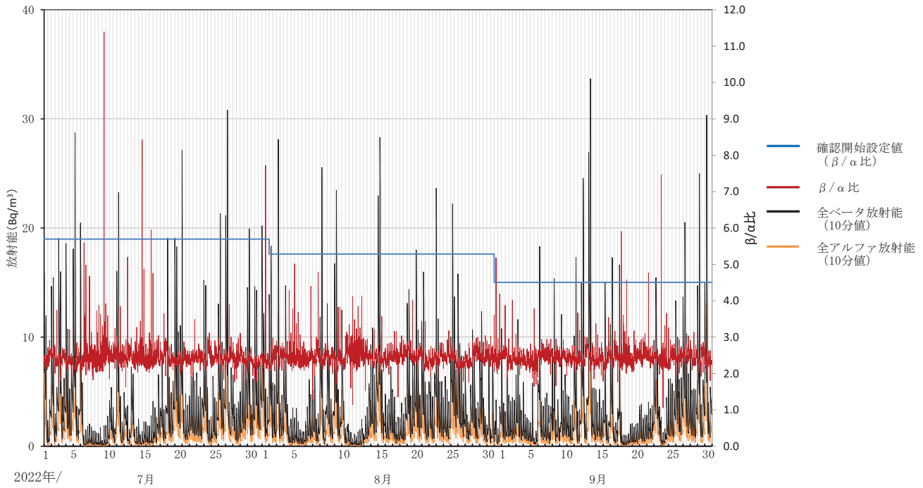
大気浮遊じん的全アルファ及び全ベータ放射能の推移（集じん中測定） 19 いわき市下桶売 （令和4年7月1日～9月30日）
