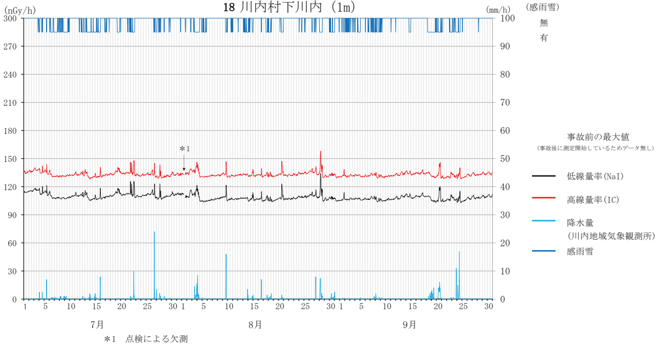
空間線量率の変動グラフ 18 川内村下川内 (1m)
