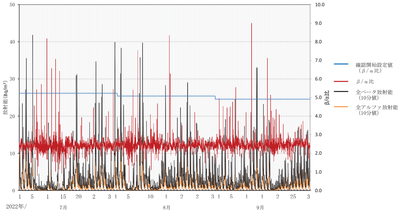
大気浮遊じんの全アルファ及び全ベータ放射能の推移（集じん中測定） 22 双葉町山田 （令和4年7月1日～9月30日）
