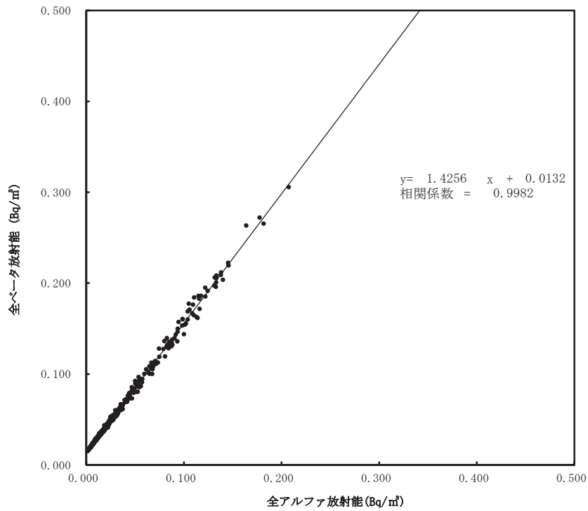
大気浮遊じんの全アルファ・全ベータ放射能の相関図 (6時間連続集じん・6時間放置後) (令和4年7月～9月) (葛尾村夏湯)
