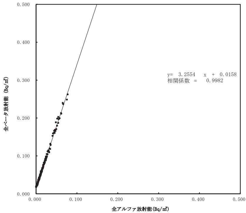
大気浮遊じんの全アルファ・全ベータ放射能の相関図 (6時間連続集じん・6時間放置後) (令和4年7月～9月) (檜葉町繁岡)
