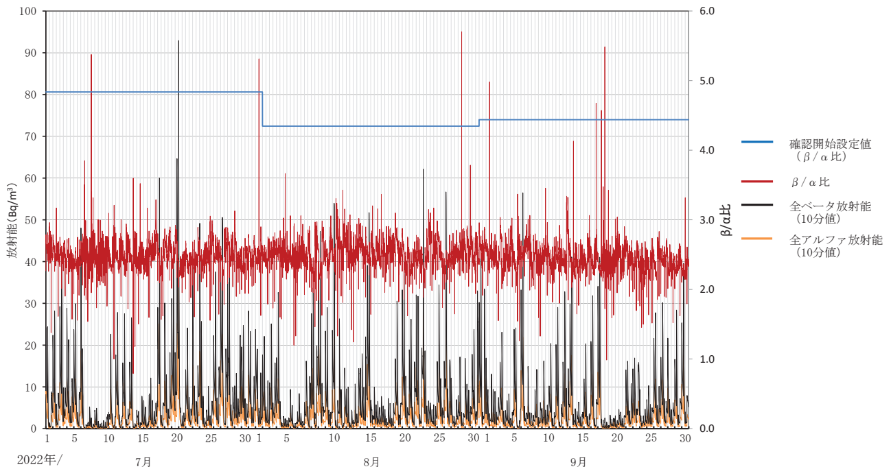
大気浮遊じん的全アルファ及び全ベータ放射能の推移（集じん中測定） 20 いわき市川前 （令和4年7月1日～9月30日）
