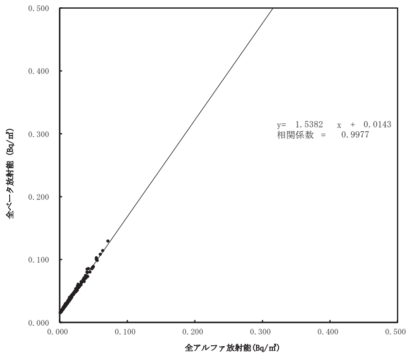
大気浮遊じんの全アルファ・全ベータ放射能の相関図 (6時間連続集じん・6時間放置後) (令和4年7月～9月) (田村市都路馬洗戸)
