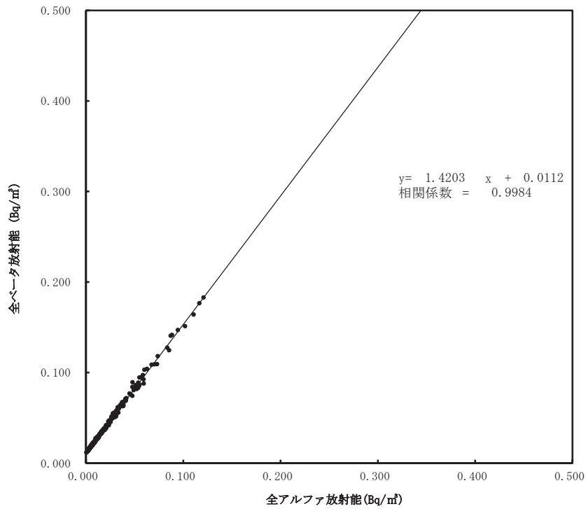
大気浮遊じんの全アルファ・全ベータ放射能の相関図 (6時間連続集じん・6時間放置後) (令和4年7月～9月) (浪江町幾世橋)
