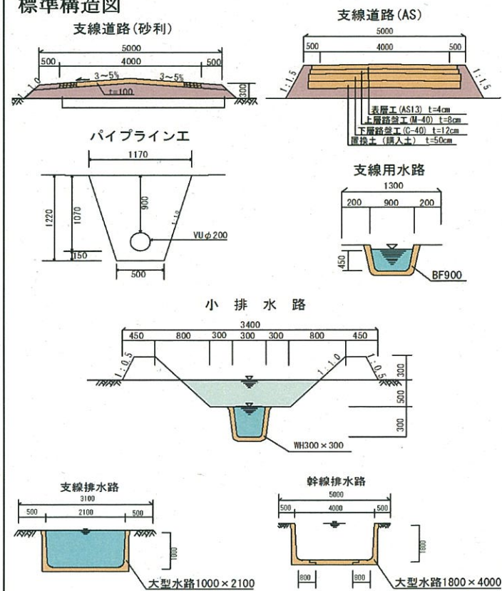
標準構造図
