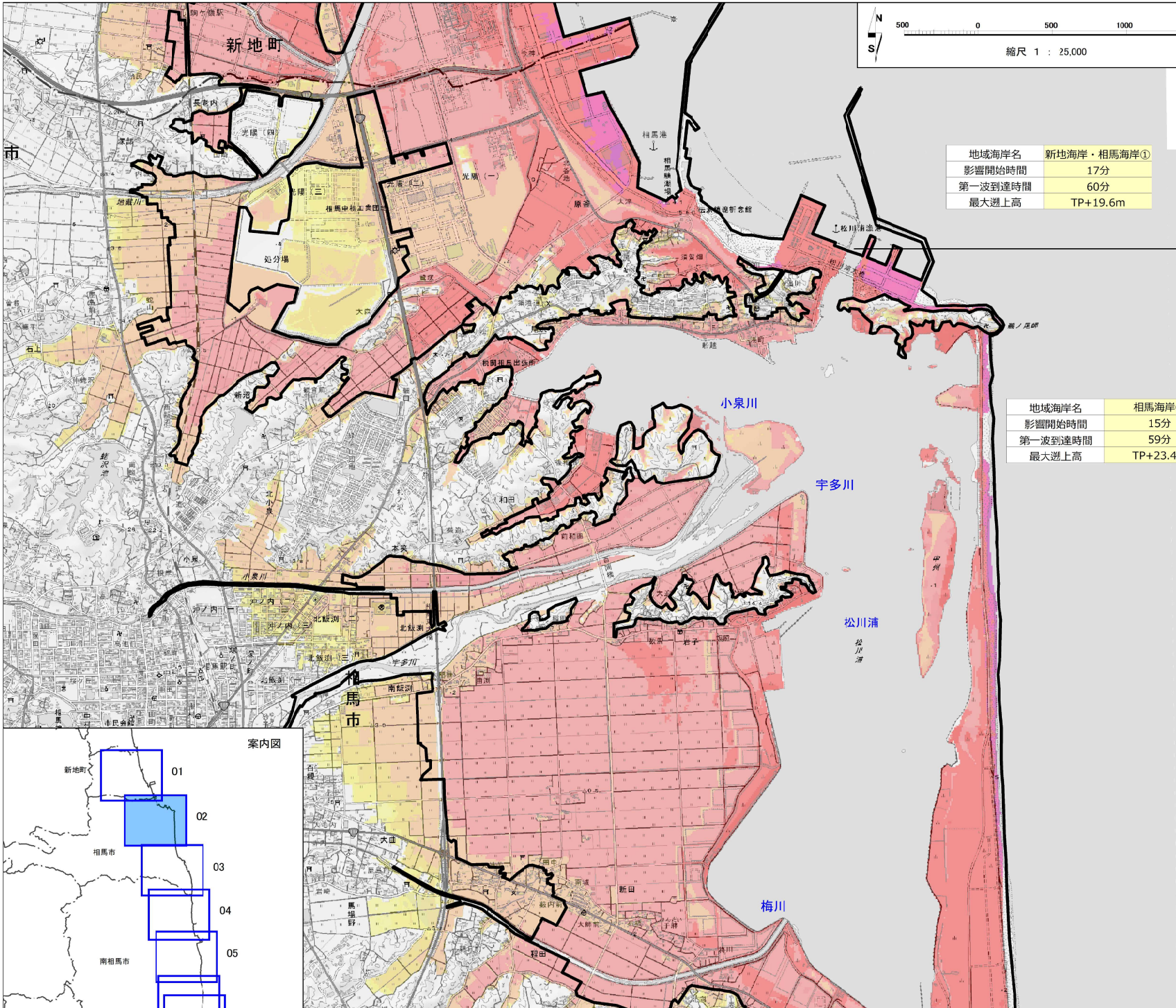
図1 最大遡上高と浸水深
