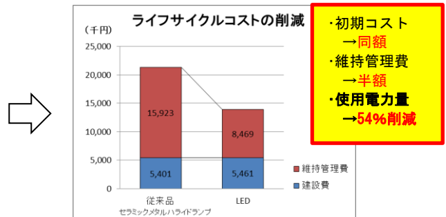
LED 事例（国道 252 号 滝トンネル（金山町））
