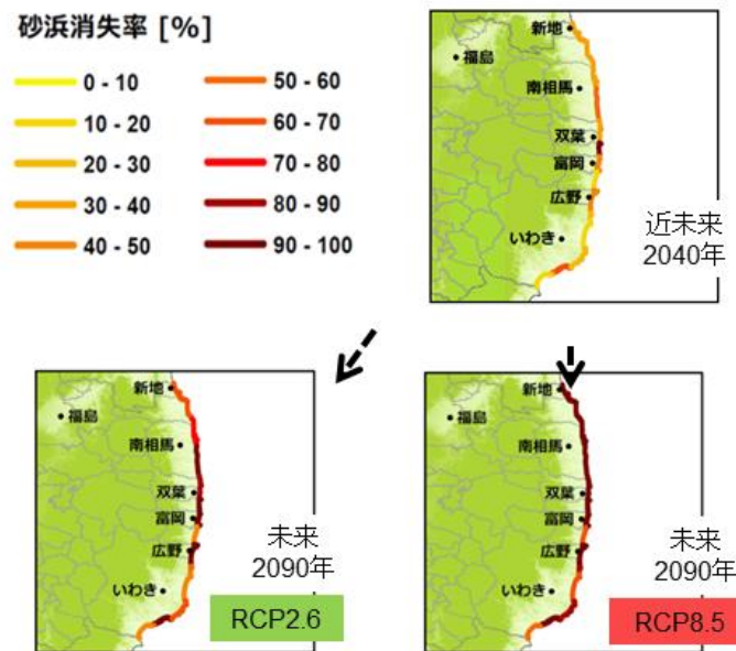
図 5-21 海面上昇による海岸侵食予測結果 現在と比較した、海岸ごとの砂浜消失率を色で示した。
