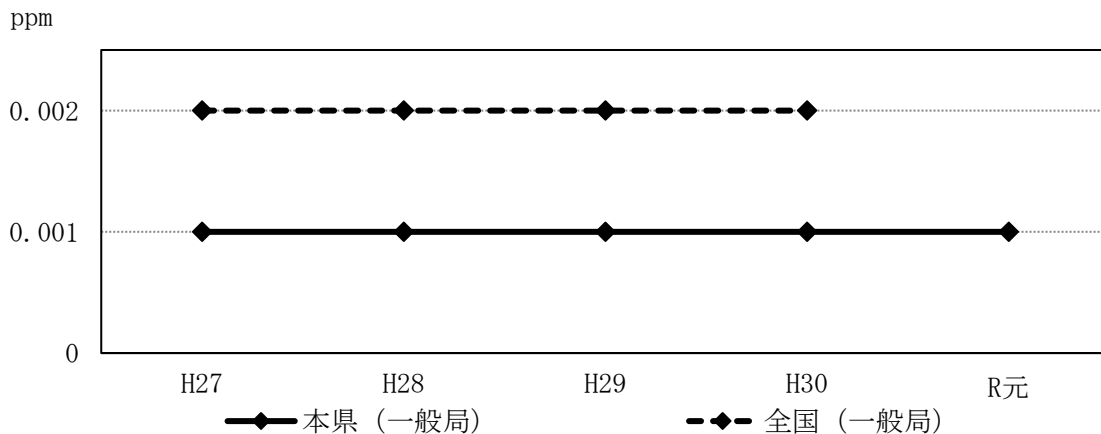
図1-1 二酸化硫黄濃度の推移
