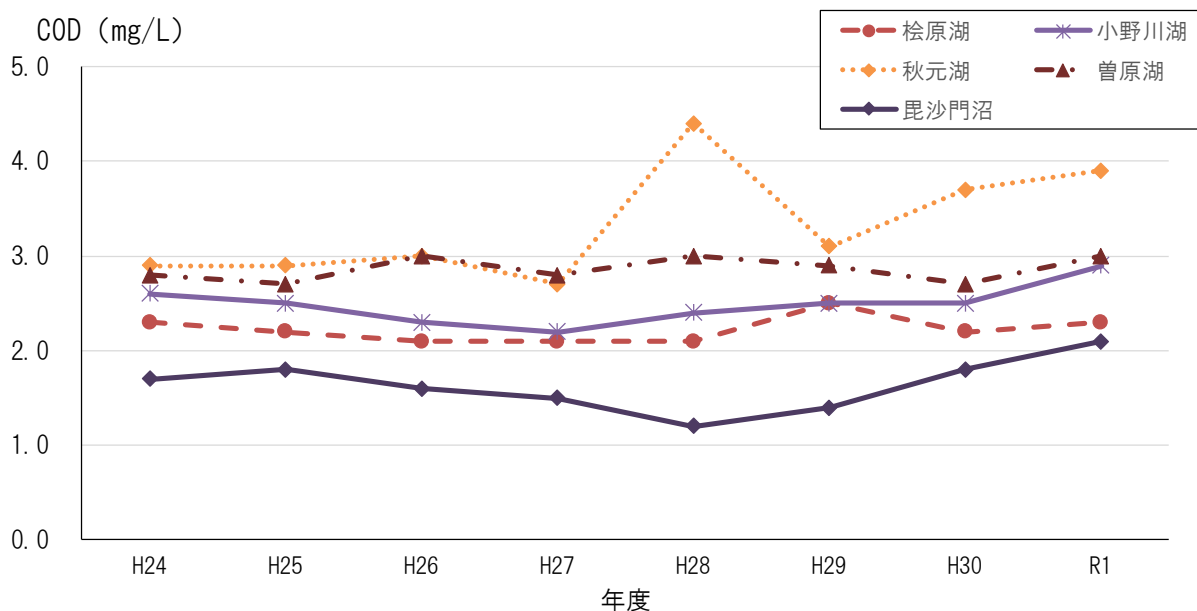
図－4 裏磐梯湖沼（湖心）におけるCOD（全層75%値）の推移
