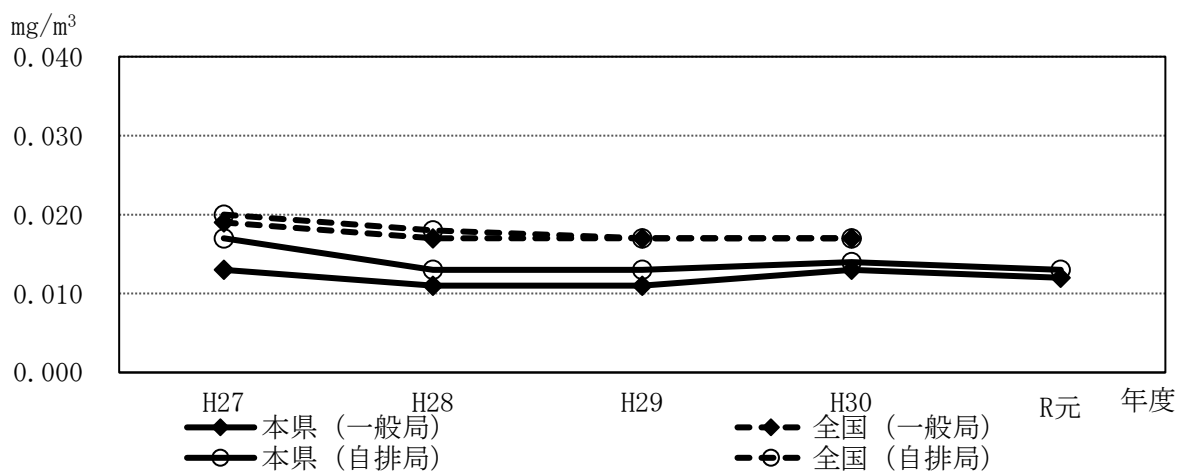
図1-3 浮遊粒子状物質濃度の推移
