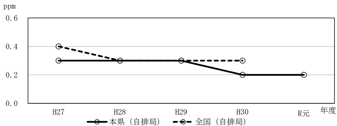
図1-2 一酸化炭素濃度の推移
