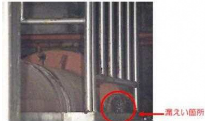
(真空破壊ラインベローズ漏えい状況：2014年調査時)
